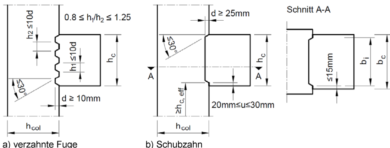
Abbildung 10: Ausbildung der Schubfuge
