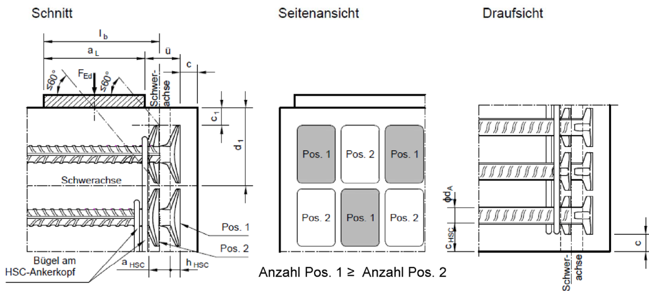
Abbildung 5: Anordnung der zweilagig gestaffelten HSC-Anker, Beispiel
