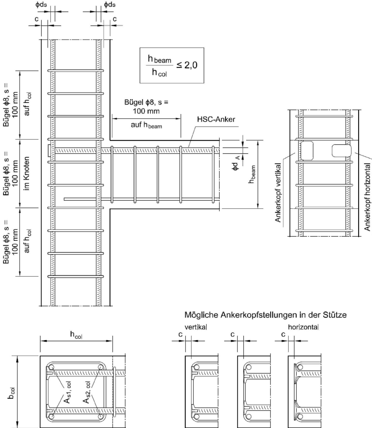
Abbildung 1: Bewehrungsführung, Beispiel
