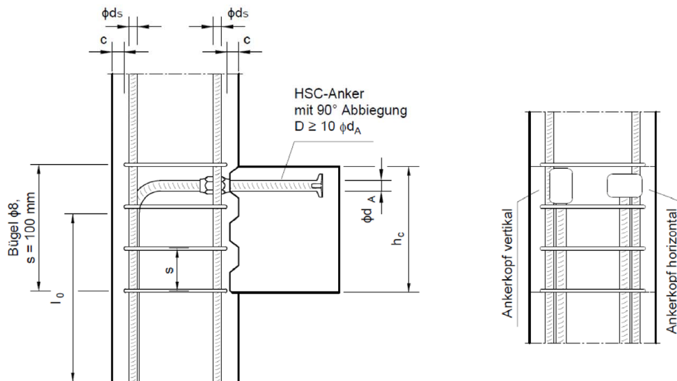
Abbildung 9: Bewehrungsführung von um 90^\circ nach unten abgelenkten HSC-Ankern in der Stütze, Beispiel
