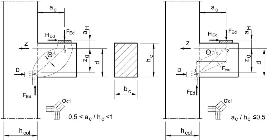
Abbildung 3: Stabwerkmodell nach DAfStb-Heft 600
