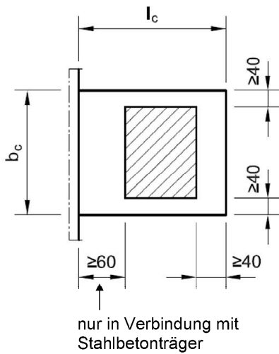
Abbildung 4: Anordnung einer Lasteinleitungsplatte, Empfehlung
