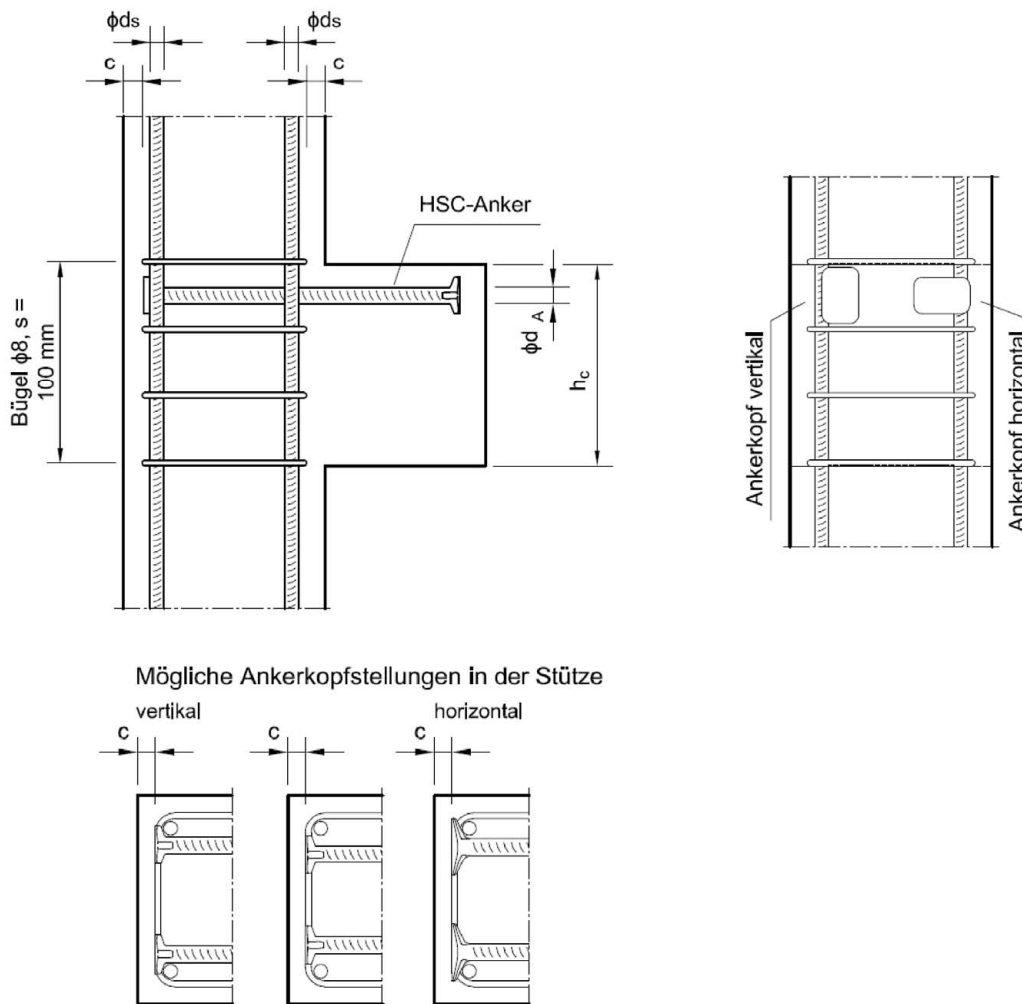
Abbildung 8: Bewehrungsführung in der Stütze, Beispiel
