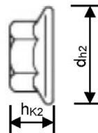
HPA-FN Sechskantmutter mit Bund, DIN EN 1661:1998-02
