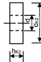
HPA-K Kopfplatte mit Innengewinde, rund. Kopfmarkierung: H 8, H A4, H HCR
