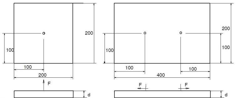
Bild 3: zentrischer Zug bzw. Querzug für einen Randabstand 100/100 mm
