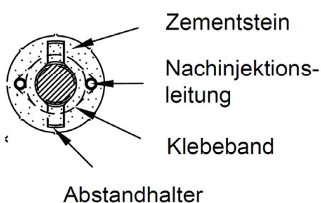
Schnitt A-A
