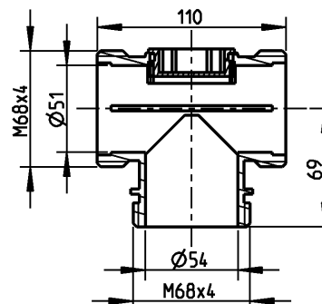
Pos. 14 T-Stück Entlüftungsleitung* Material: PA6
