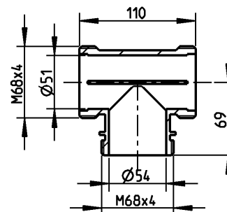
Pos. 10 T-Stück Entlüftungsleitung Material: PA6
