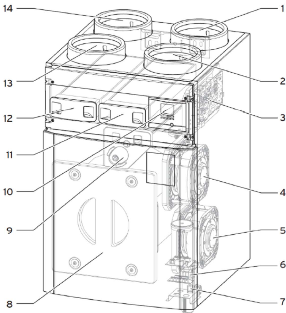
Lufttechnischer Aufbau des recoVAIR Lüftungsgerätes
