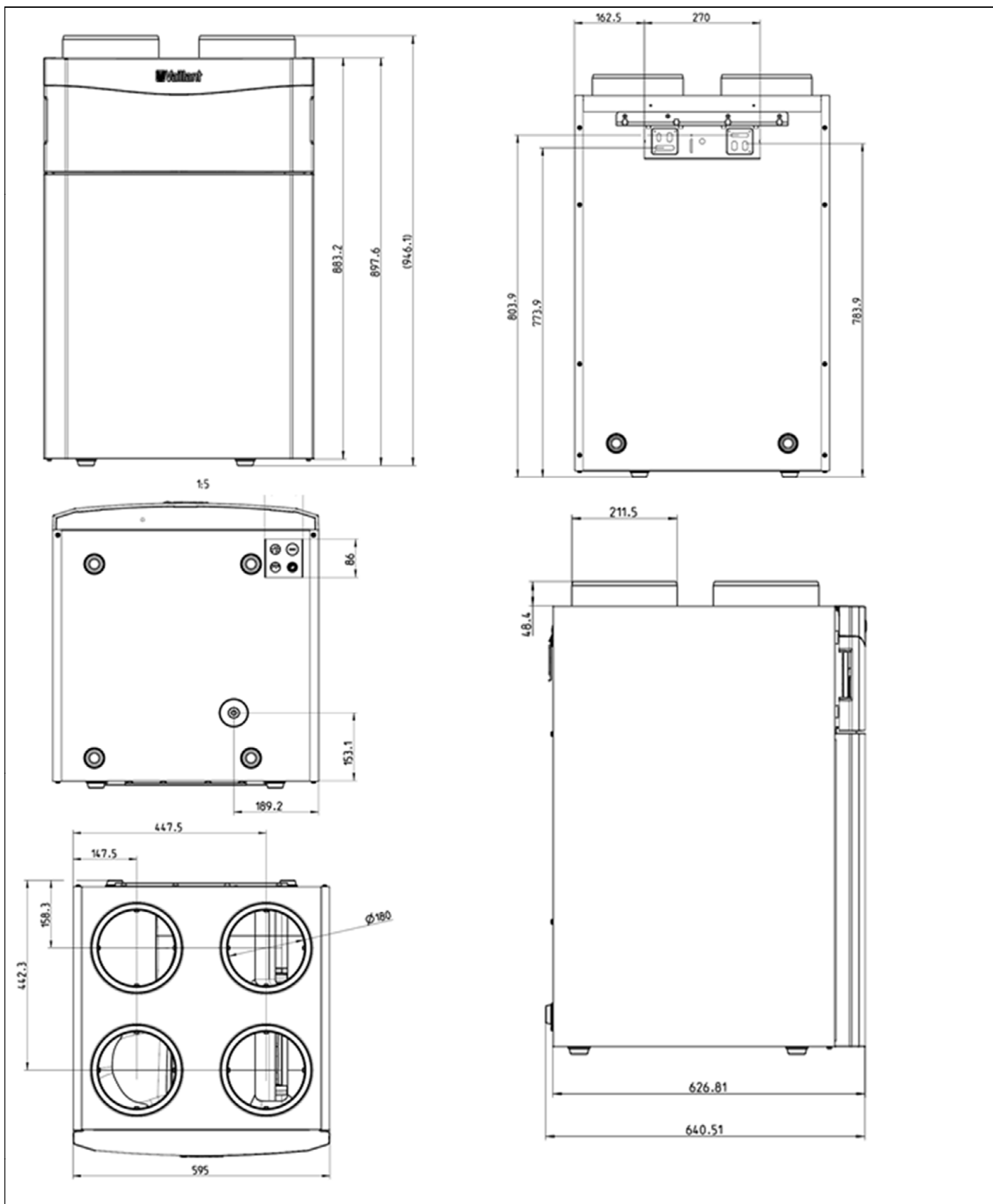
Zentrales Lüftungsgerät mit Wärme- und Feuchterückgewinnung Typ "recoVAIR - VAR 360/4 E"
