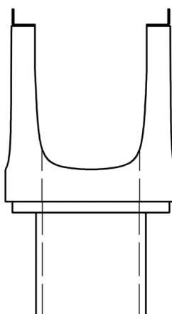
Schnitt A-A
