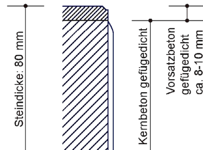
Schnitt (Randausschnitt)
