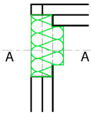
Detailschnitt B-B
