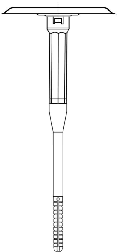
Zahn ZCTS-Tülle 4,8 mit ZCTS-Teller und Dübelverlängerung
