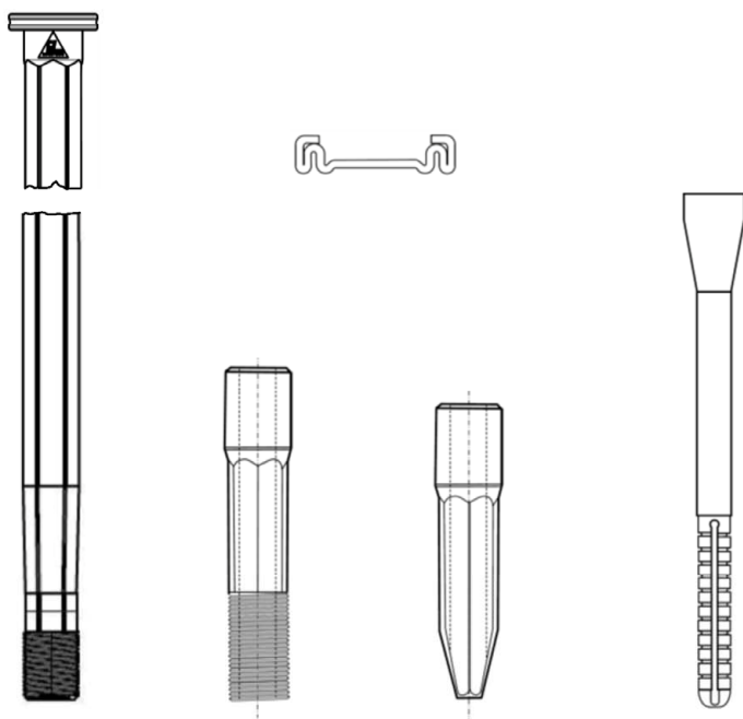
Zahn ZSSB-Modul-Tülle 4,8 mit Modul, Vorsatzdübel und Schiene
