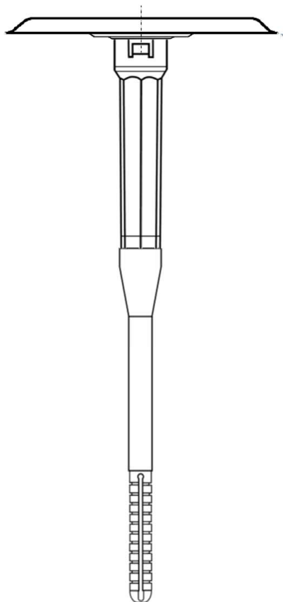
Zahn ZCTS-Tülle 4,8 mit ZCTS Teller und Vorsatzdübel
