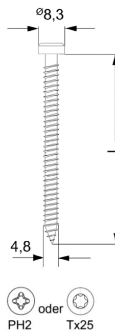
Zahn ZDBK Dübel 4,8 x L
