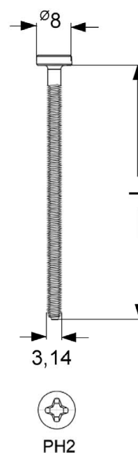
Zahn Metrische Schraube E 3,14 x L
