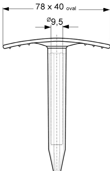
Zahn ZHRD oval mit Spreizdübelverlängerung
