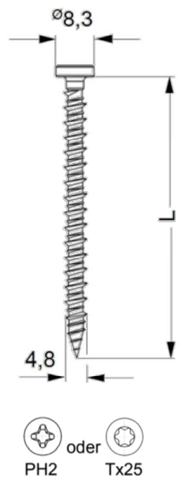
Zahn ZHBK 4,8 x L
