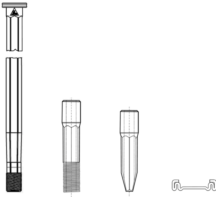
Zahn ZSSB-Modul-Tülle mit Modul 6,0 und Schiene
