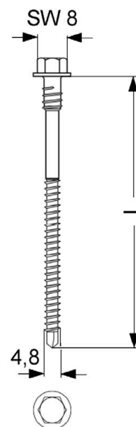
Zahn ZDBS-VB 4,8 x L
