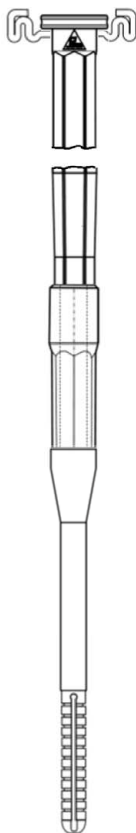
Zahn ZSSB-Modul-Tülle 4,8 mit Modul, Vorsatzdübel und Schiene
