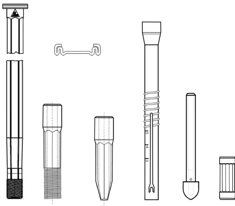
Zahn ZSSB-Modul-Tülle 4,8 mit Modul, Spreizdübelverl. und Schiene
