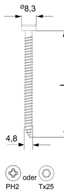
Zahn ZDBK Dübel 4,8 x L
