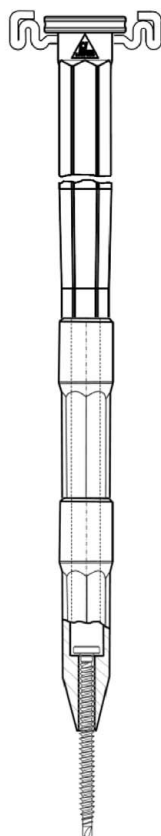
Zahn ZSSB-Modul-Tülle mit Modul 4,8 und Schiene
