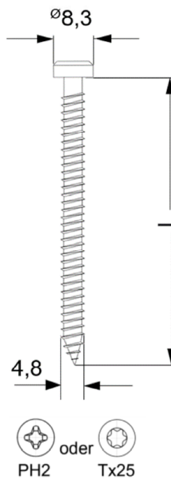
Zahn ZDBK Dübel 4,8 x L
