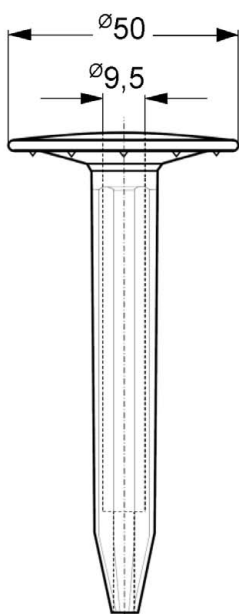
Zahn ZKSH grau / rund
