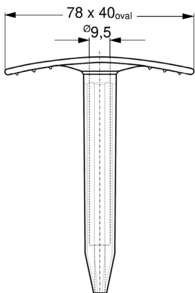
Zahn ZKSH oval mit Dübelverlängerung
