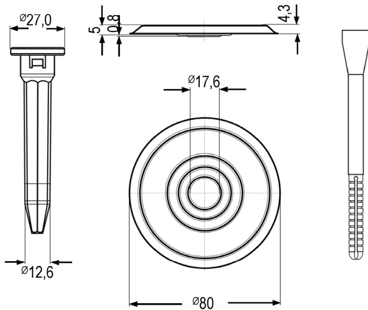
Zahn ZCTS-Tülle 4,8 mit ZCTS-Teller und Dübelverlängerung
