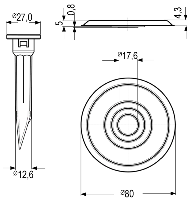
Zahn ZCTSplus-VB mit Pfahlspitzen-Tülle 4,8 mit ZCTS-Teller
