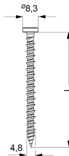
Zahn ZHBK-E 4,8 x L
