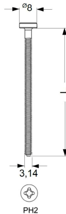
Zahn Metrische Schraube E 3,14 x L
