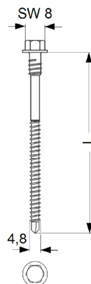
Zahn ZDBS-E 4,8 x L
