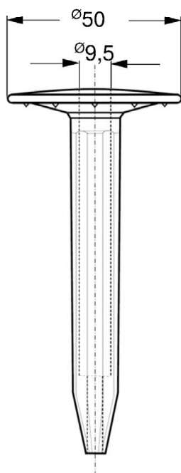
Zahn ZKSH rund mit Dübelverlängerung
