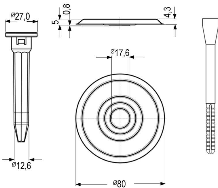
Zahn ZCTS-Tülle 4,8 mit ZCTS Teller und Vorsatzdübel
