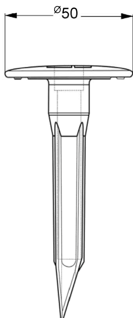
Zahn ZKSH-Rplus Pfahlspitze
