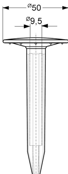
Zahn ZHRD rund mit Spreizdübelverlängerung
