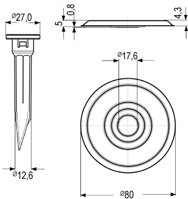
Zahn ZCTSplus mit Pfahlspitzen-Tülle 4,8 mit ZCTS-Teller
