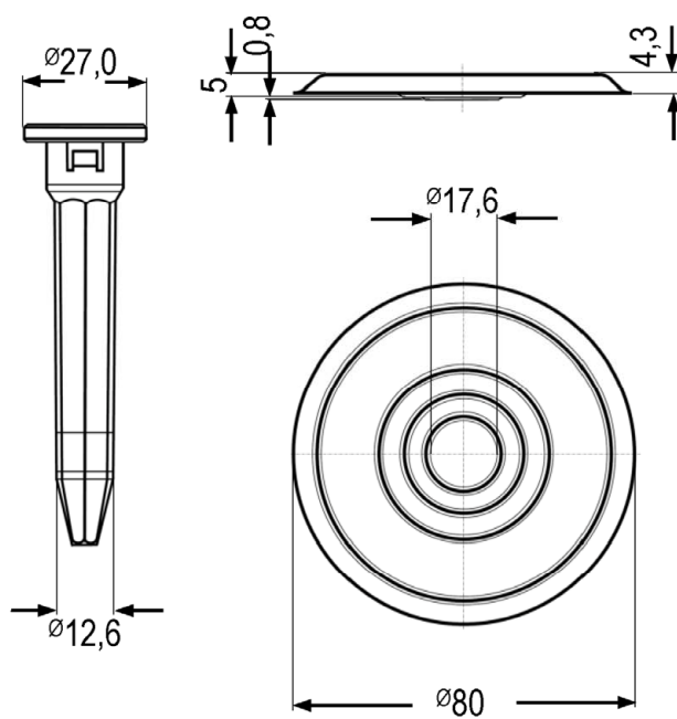
Zahn ZCTS-Tülle 6,0 mit ZCTS-Teller
