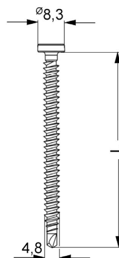
Zahn ZDBK 4,8 x L
