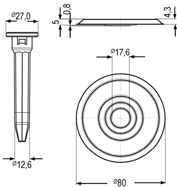
Zahn ZCTS-Tülle 6,0 mit ZCTS-Teller
