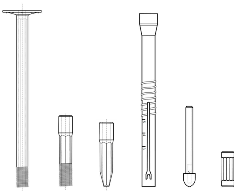
Zahn ZKSK rund Modul 4,8 mit Spreizdübel
