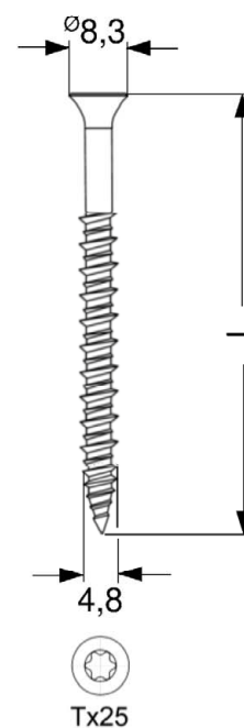
Zahn ZHBK-E TK 4,8 x L
