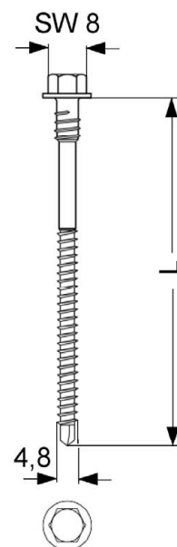
Zahn ZDBS-E 4,8 x L
