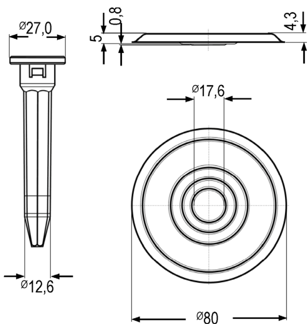
Zahn ZCTS-Tülle 4,8 mit ZCTS-Teller
