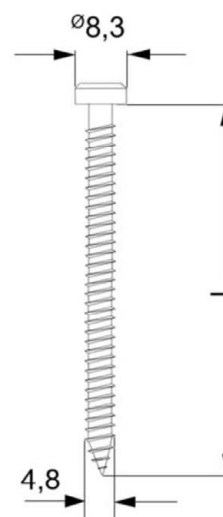
Zahn ZDBK Dübel 4,8 x L
