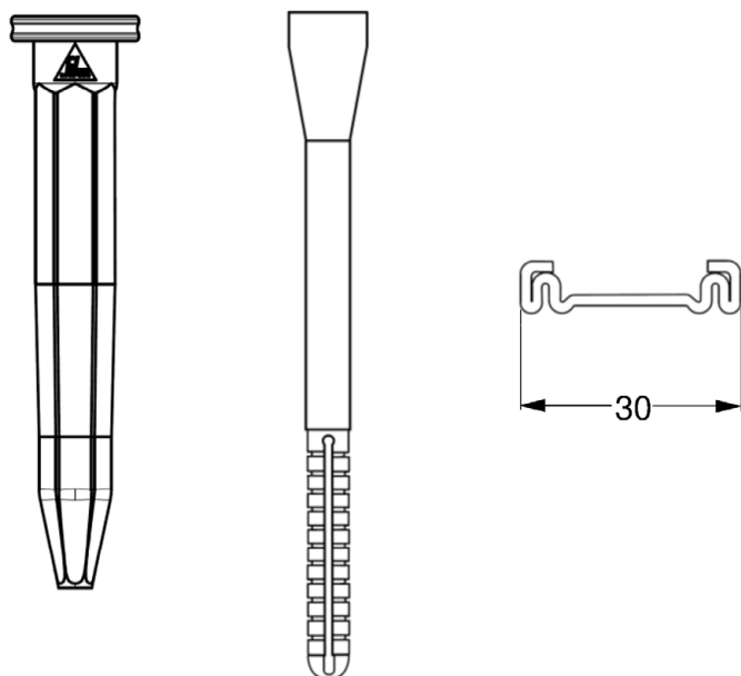
Zahn ZSSB-Tülle 4,8 mit Vorsatzdübel und Schiene
