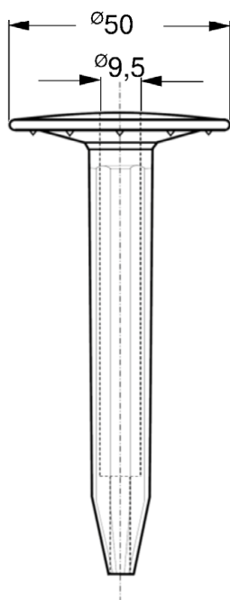
Zahn ZKSH rund
