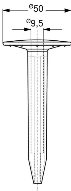
Zahn ZKSH grau / rund
