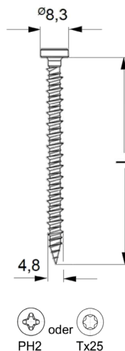
Zahn ZHBK-E 4,8 x L
