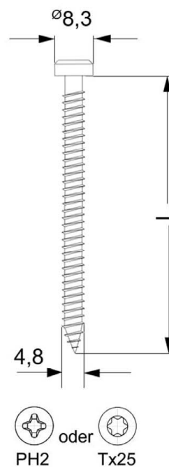
Zahn ZDBK Dübel 4,8 x L
