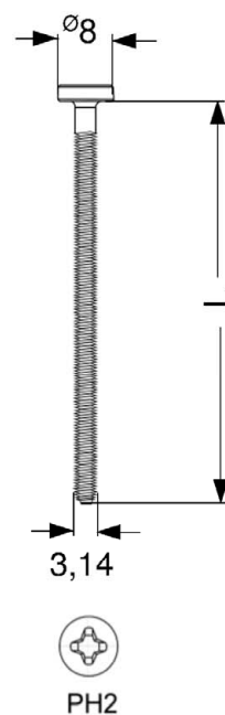
Zahn Metrische Schraube E 3,14 x L
