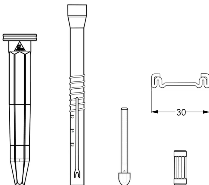
Zahn ZSSB-Tülle 4,8 mit Spreizdübelverl. und Schiene
