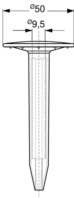
Zahn ZKSH rund
