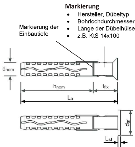
Dübelhülse KT 14
