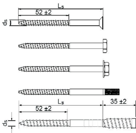
Spezialschraube KT 10
