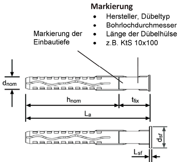
Dübelhülse KT 10
