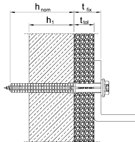
Einbauszustand SDF-10H in einer Wetterschale ( h_{nom} ) Kopfform: Kragenkopf mit Bund (KB)
