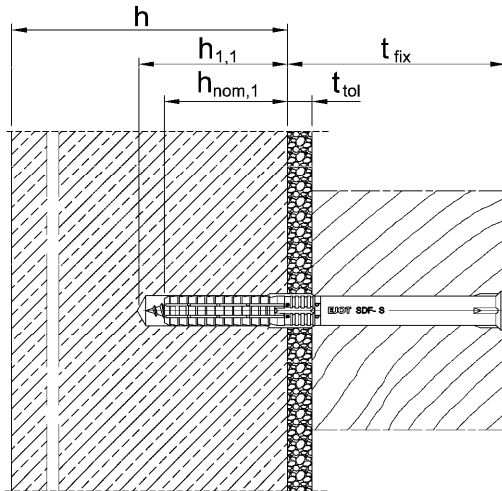
Einbauszustand SDF-10V in Beton ( h_{nom1} ) Kopfform: Senkkopf (S)
