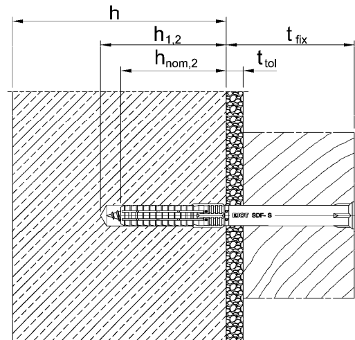
Einbauszustand SDF-10V in Vollstein ( h_{nom2} ) Kopfform: Senkkopf (S)
