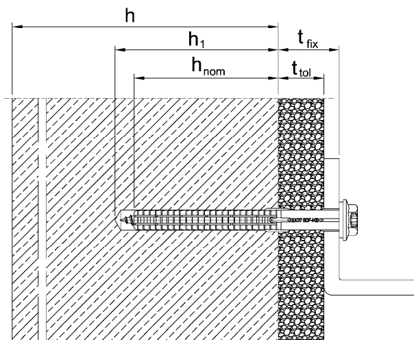
Einbauszustand SDF-10H in Beton/Mauerwerk/ Porenbeton ( h_{nom} ) Kopfform: Kragenkopf mit Bund (KB)
