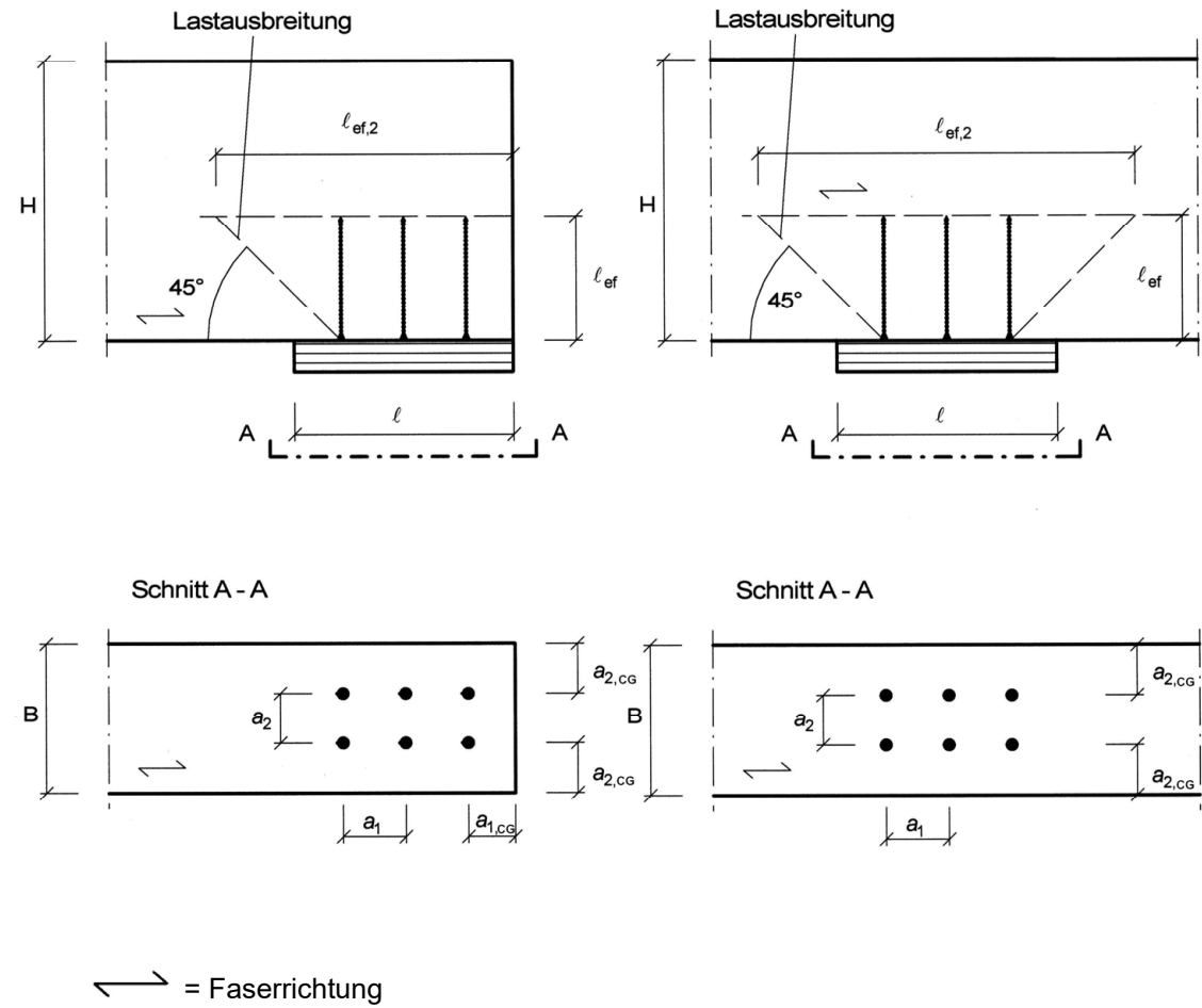
Abbildung A.3.1 Verstärktes Endauflager (links) und verstärktes Zwischenaufleger (rechts)
