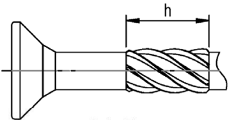
Schaftfräser
