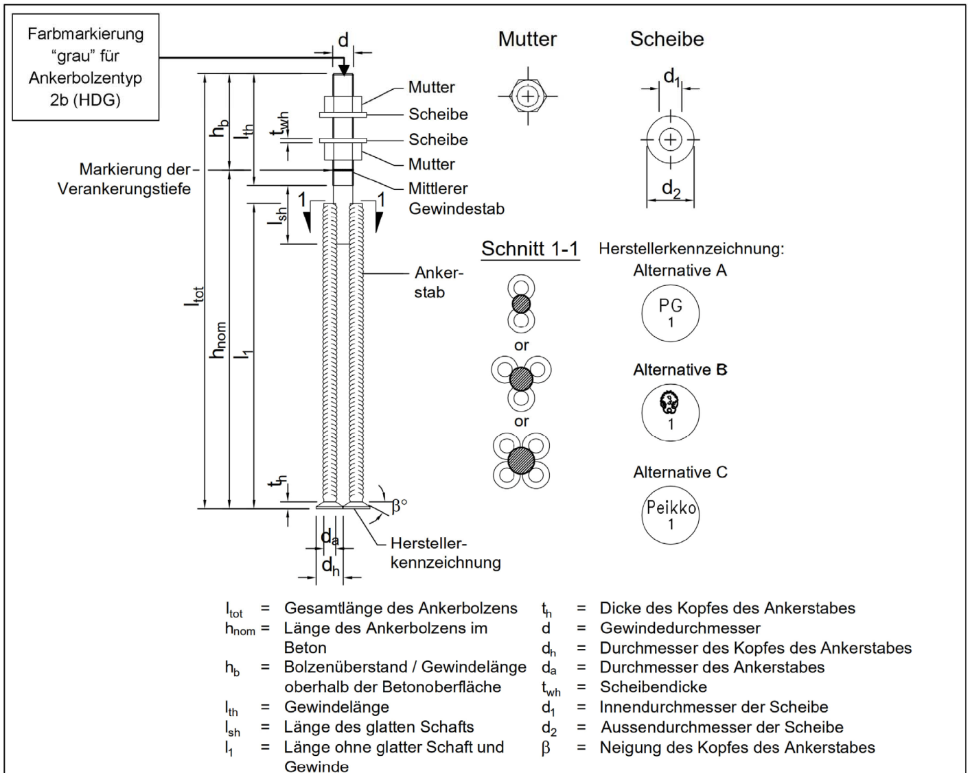
Abbildung 3. Abmessungen der PPM® L Ankerbolzen
