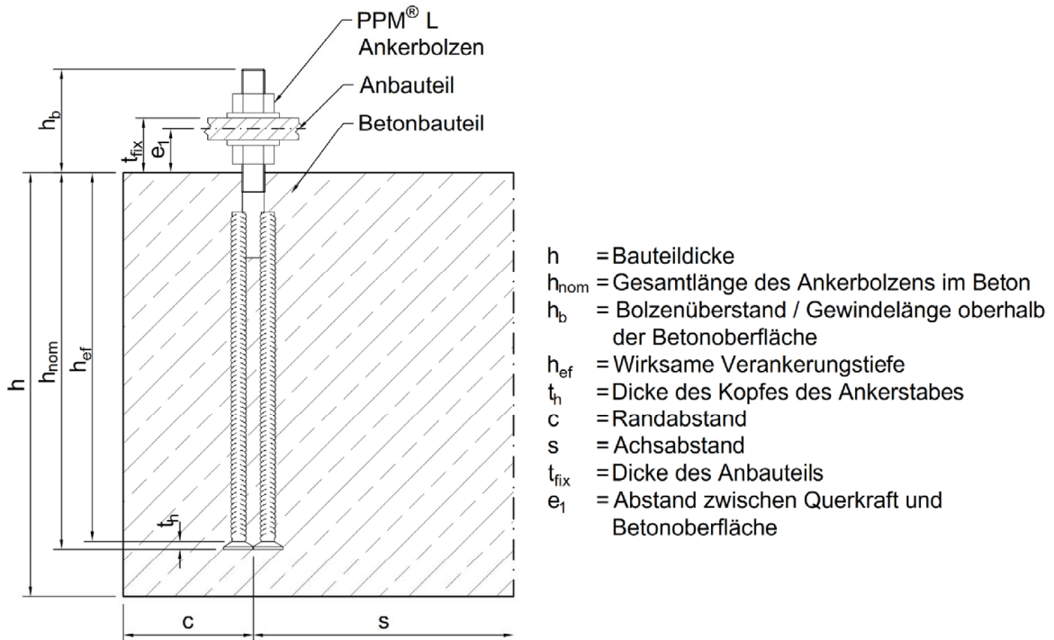
Abbildung 2. (b) Stahl-Stahl-Kontakt
