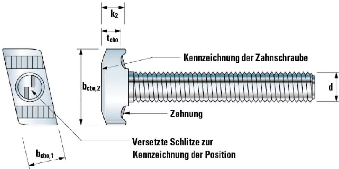
Zahnschraube FBC-S-225
