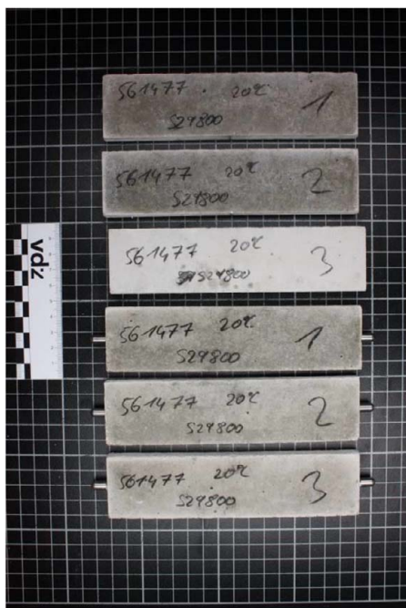
Bild A2: Probekörper mit CEM III/B 32,5 N-LH/SR nach der Sulfatlagerung; Links: nach 182 Tagen bei 20 °C; Rechts: nach 91 Tagen bei 5 °C
