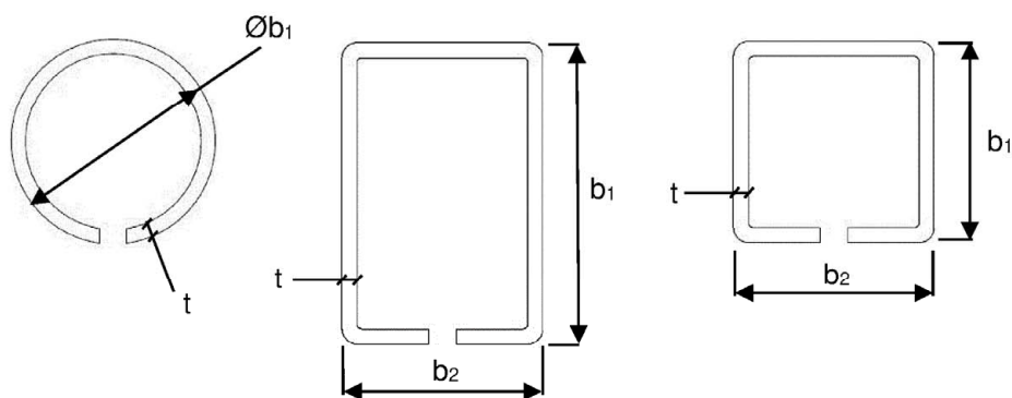
Hohlprofil geschlitzt
