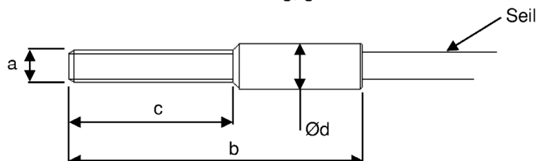
Gwindefitting, gehämmert
