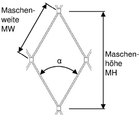
Maschengeometrie
