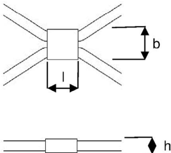
Netzklemme verpresst
