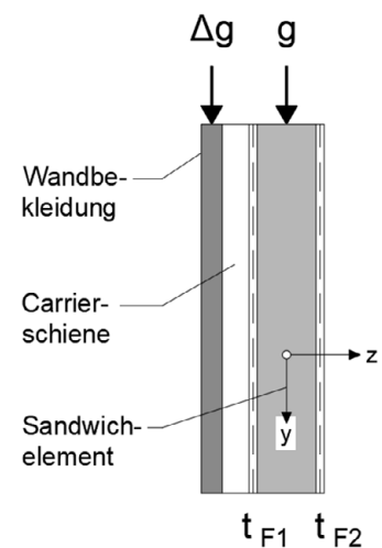
Schnitt C-C
