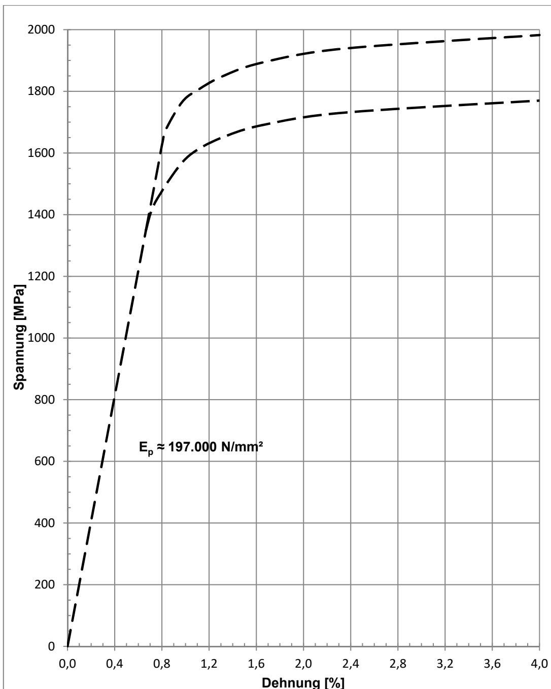
Bild 2: Prinzipieller Spannungs-Dehnungs-Linie-Verlauf
