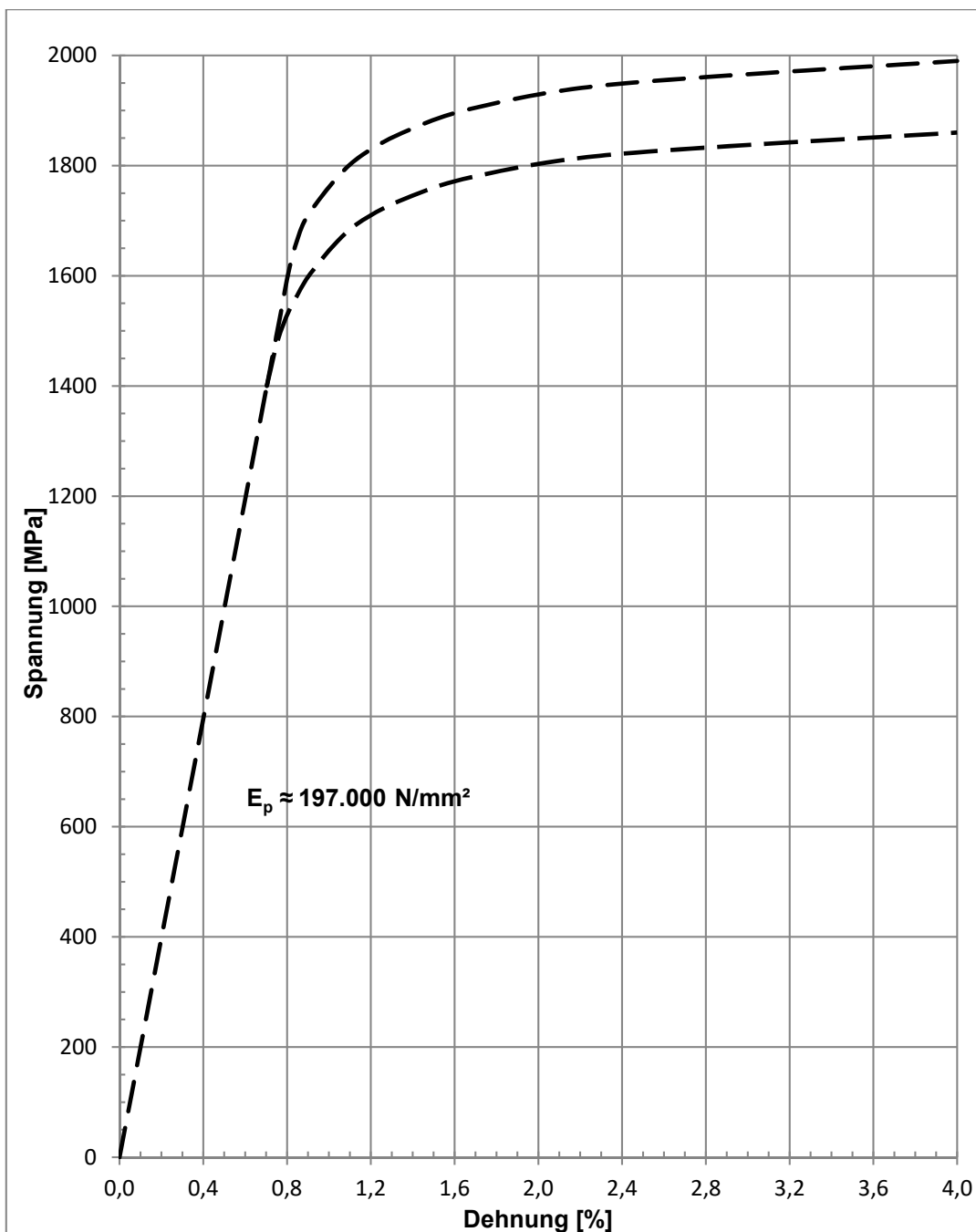
Bild 2: Prinzipieller Spannung-Dehnungs-Linie-Verlauf
