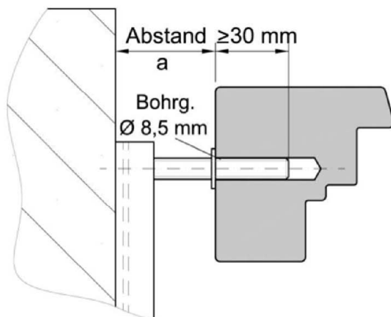
Einbau Holz – Fensterprofile
