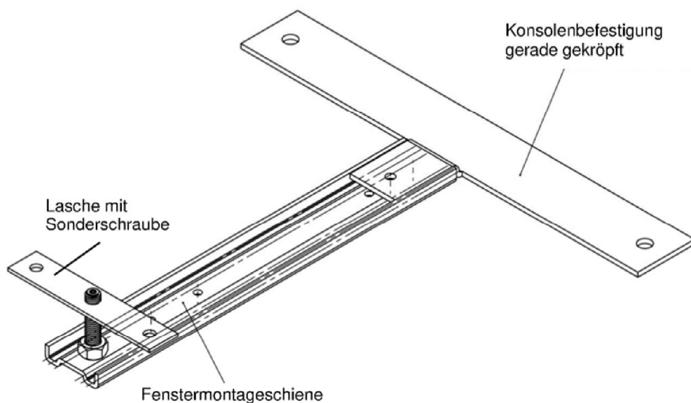
Fenstermontageschiene mit Konsolenbefestigung gerade gekröpft
