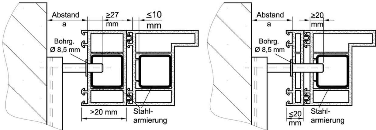
Einbau PVC – Profile mit Stahlarmierung □ - oder U – Form, t \geq 1,5 mm
