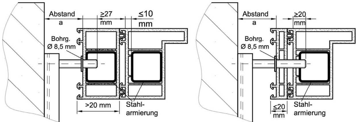
Einbau PVC – Profile mit Stahlarmierung □ - oder U – Form, t \geq 1,5 \text{ mm}
