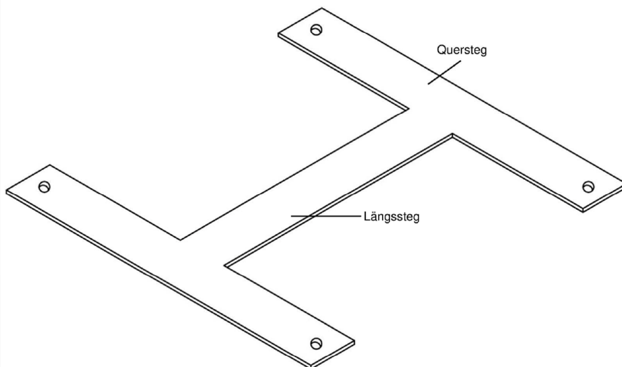
H – Konsole gerade (ohne Fenstermontageschiene dargestellt)
