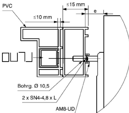
PVC mit Verbreiterung nicht armiert
