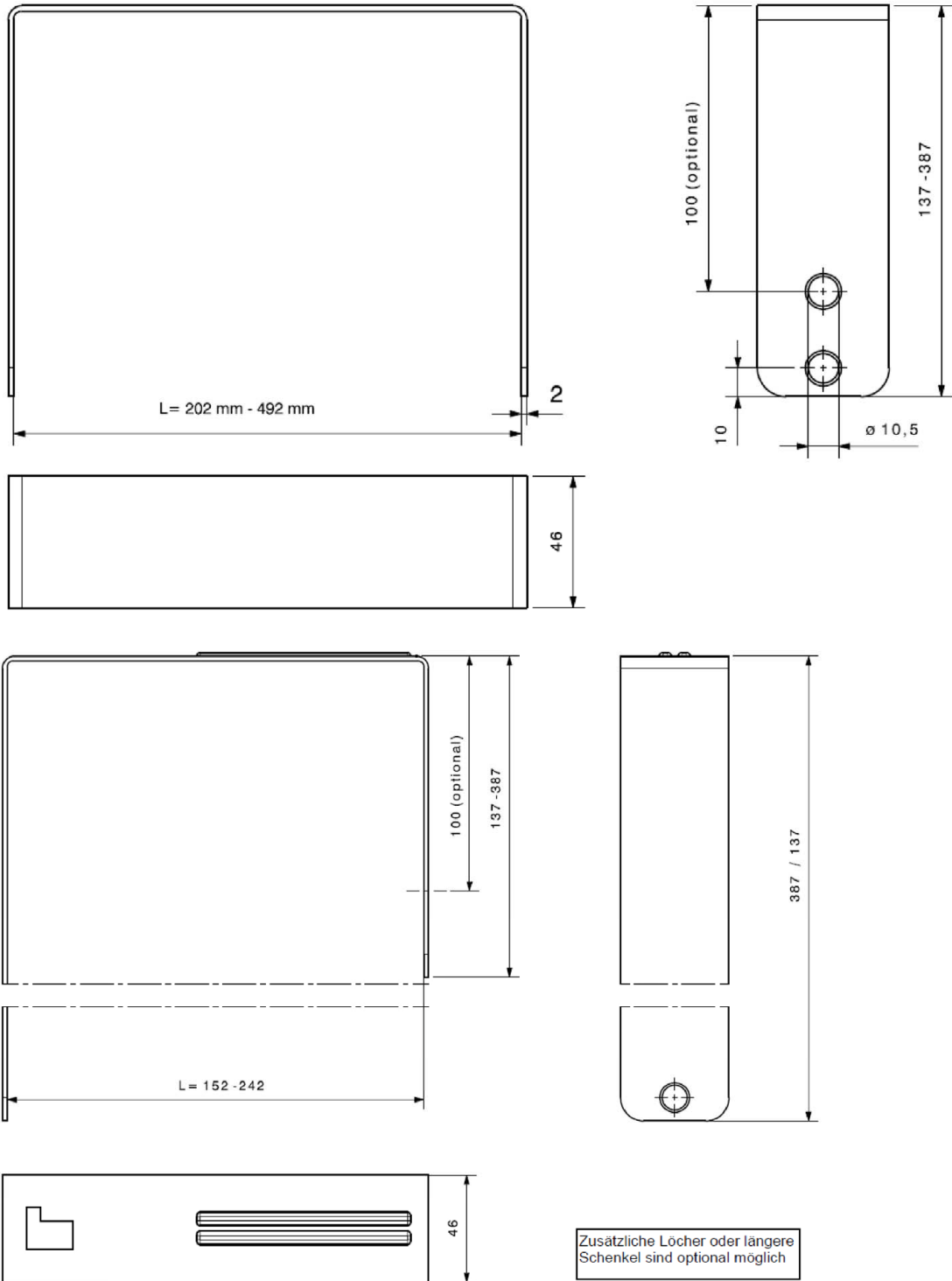
Mauerwerksklemme, Varianten seitlich
