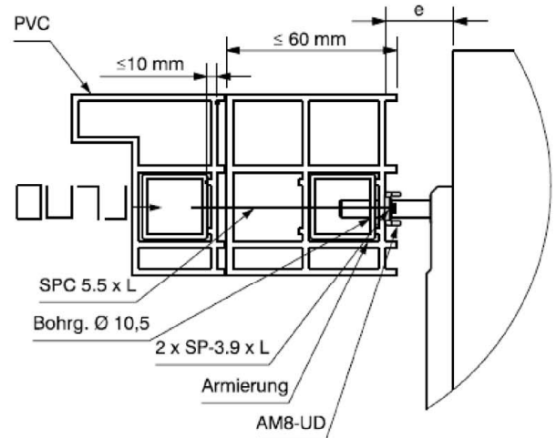
PVC mit Verbreiterung armiert
