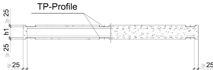
Schnitt B-B
