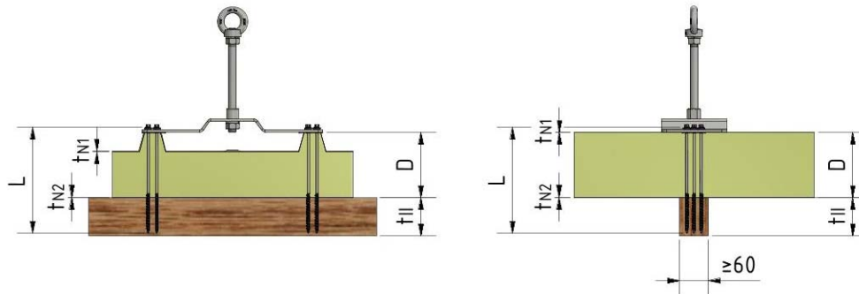
Abbildung 3a - Beispiel für die Ausführung auf Holzpfeife
