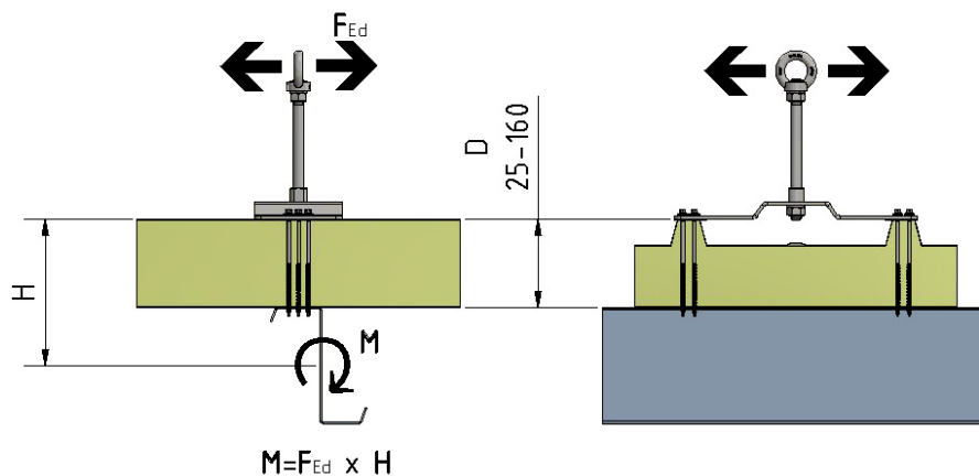
Abbildung 4 - Einwirkungen für die Unterkonstruktion für Lastfall Absturz (Beispiel)
