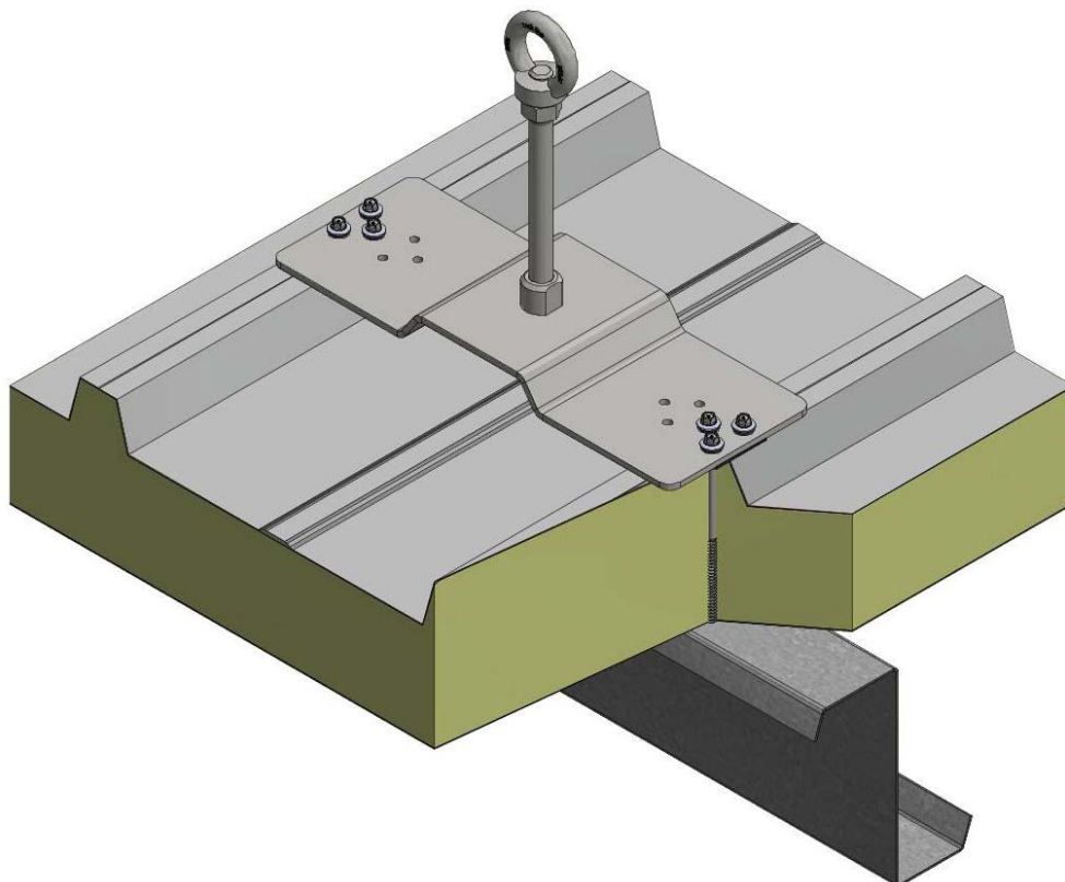
Abbildung 1 - schematische Darstellung der Befestigung
