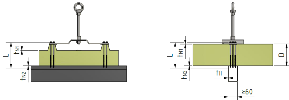
Abbildung 3c - Beispiel für die Ausführung mit Hohlprofilen als Pfeife ( 3\text{mm} \leq t_{II} \leq 12\text{mm} )
