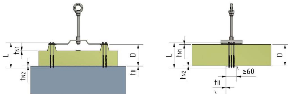
Abbildung 3b - Beispiel für die Ausführung auf Stahl-Z-Pfeife ( t_{II} = 2 und t_{II} = 4 mm)
