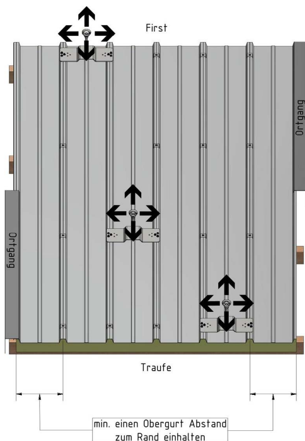
Abbildung 2 - Montagevorgaben für die Planung der Anschlageinrichtungen
