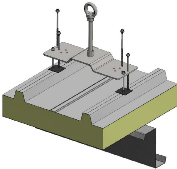
Abbildung 5 - Abdichtung Anschlagseinrichtung zu Sandwichelement
