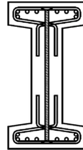
Beispiel 5: I - Träger
