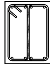
Beispiel 6: Kompakt- querschnitt (Balken bzw. Plattenbalken)
