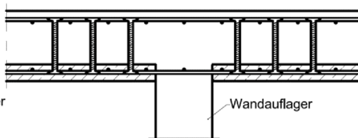
Beispiel 7: Stahlbetonwände, z.B. im Bereich von Öffnungen
