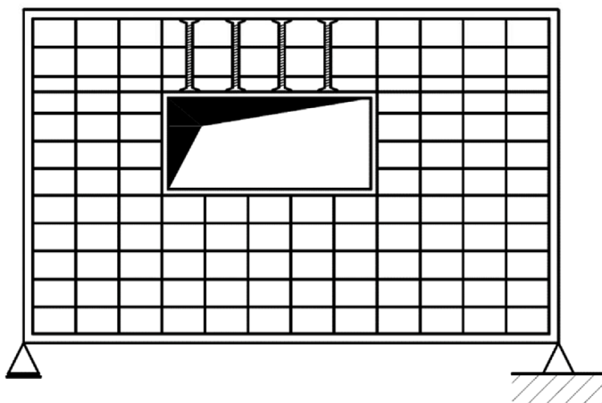
Beispiel 7: Stahlbetonwände, z.B. im Bereich von Öffnungen
