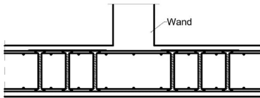
Beispiel 2: Bodenplatte Einbau von oben
