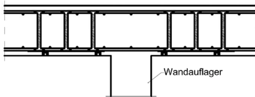
Beispiel 1: Deckenplatte Einbau von unten
