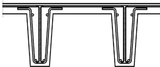
Beispiel 6: Kompakt- querschnitt (Balken bzw. Plattenbalken)
