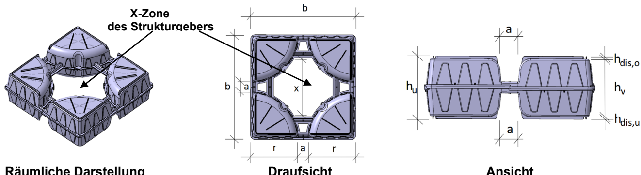
Bild 1: Strukturgeber (Rippenhöhe oben u. unten = 10 mm) und Darstellung der X-Zone
