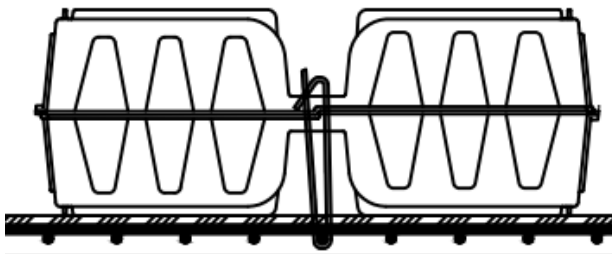
Bild 7: Befestigung der COBIAX CLS-Einbauelemente untereinander
