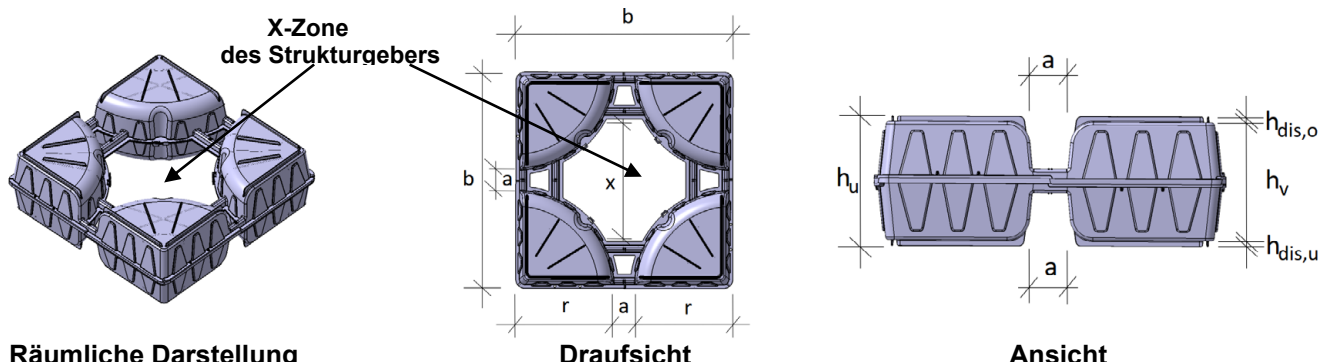
Bild 2: Strukturgeber (Rippenhöhe oben u. unten = 15 mm) und Darstellung der X-Zone
