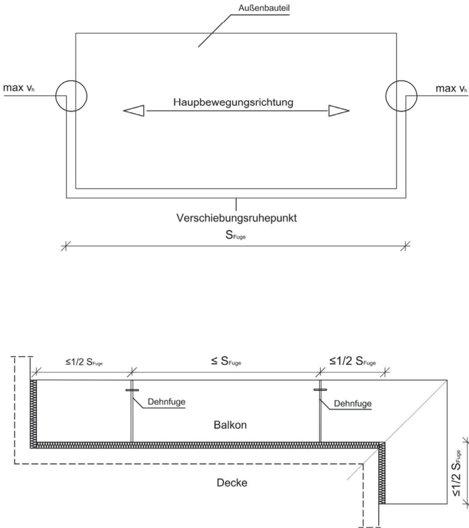
Zulässige Fugenabstände s_{Fuge} in [m]
