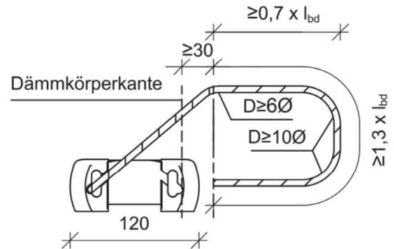
- Variante mit abgebogenen Querkraftstäben
