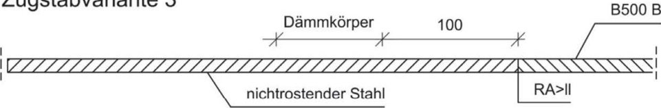
Zugstabvariante 3
