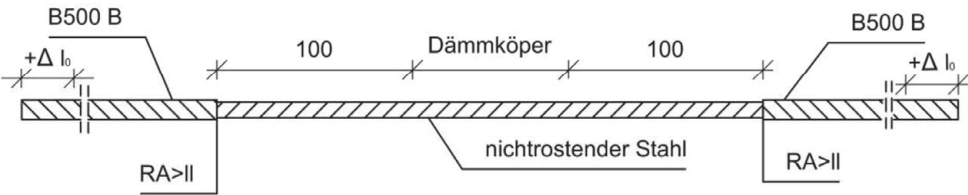
Zugstabvariante 3
