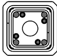
Bewehrung Stütze
