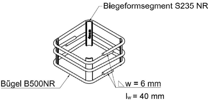
Isometrie
