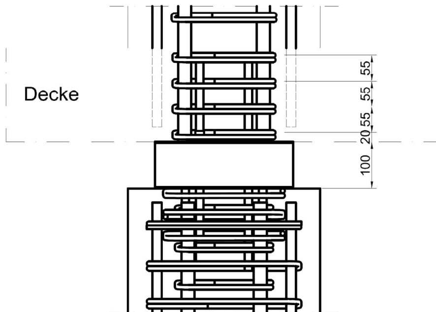
Anschluss mit Decke und Stütze oberhalb
