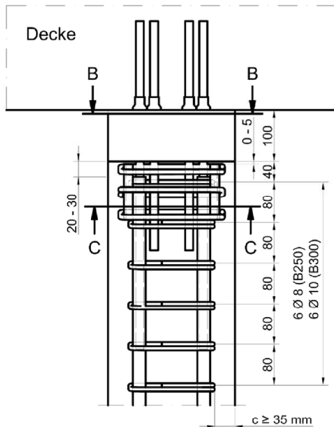
Bewehrung Stütze
