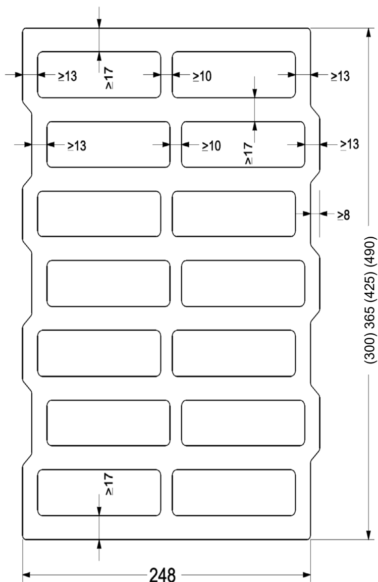
Alternative Stirflächenausbildung unter Einbehaltung der Mindeststegdicken möglich
