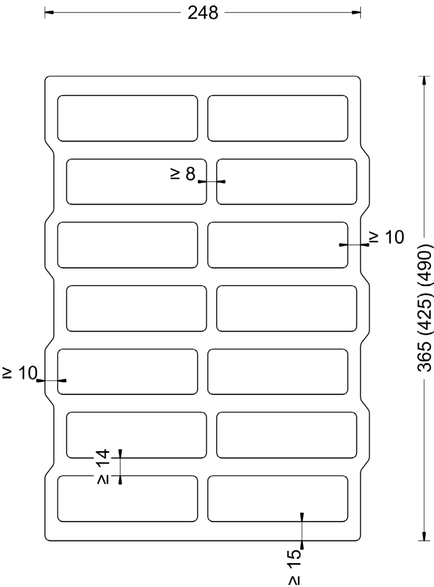
Alternative Stirnflächenausbildung unter Einbehaltung der Mindeststegdicken möglich
