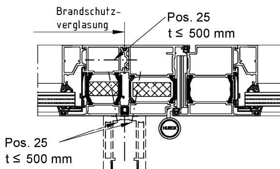
Schnitt D 1
