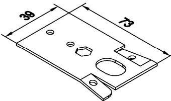
Z 917384 Montagehalter, Edelstahl in Profalnute eindrehen und mit Senkbohrschraube Z 911050 sichern
