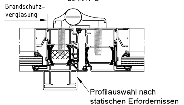
Schnitt D
