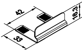
Z 917537 Sicherungswinkel für Glasleisten, Edelstahl für Glasstärke 28 - 35 mm nur in Verbindung: CONTRAFLAM 30 und runder Glasleiste
