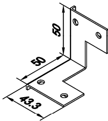
Z 996412 Eckwinkel, Edelstahl für Füllungsgewichte \geq 180 kg
