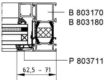
Verglasung von außen
