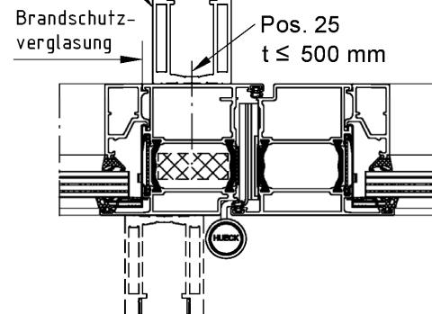
Schnitt D 1
