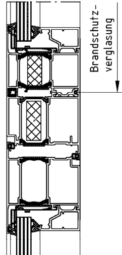
Schnitt E 1
