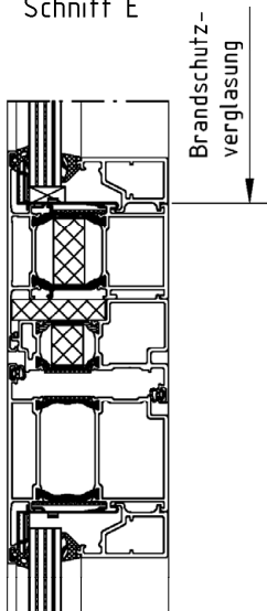
Schnitt E
