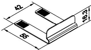
Z 917860 Sicherungswinkel für Glasleisten, Edelstahl für Glasstärke 48 - 56 mm nur in Verbindung: CONTRAFLAM 30 und runder Glasleiste
