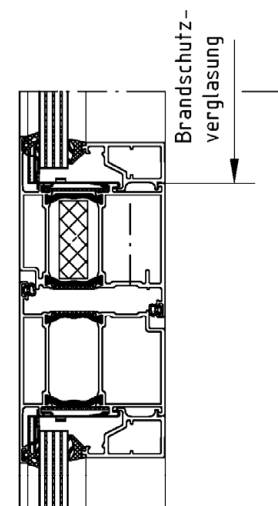
Schnitt E 1
