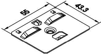
Z 917856 Glashalter für Verglasung von aussen
