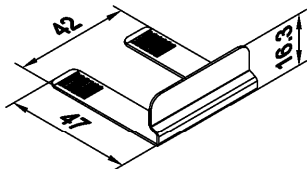
Z 917855 Sicherungswinkel für Glasleisten, Edelstahl für Glasstärke 35 - 48 mm nur in Verbindung: CONTRAFLAM 30 und runder Glasleiste
