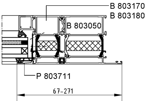
Verglasung von außen
