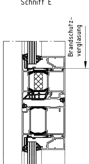
Schnitt E
