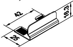
Z 917277 Sicherungswinkel für Glasleisten, Edelstahl für Glasstärke 13 - 28 mm nur in Verbindung: CONTRAFLAM 30 und runder Glasleiste
