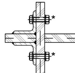
Schnitt 5.1.2.3
