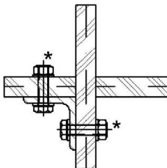
Schnitt 5.1.2.4
