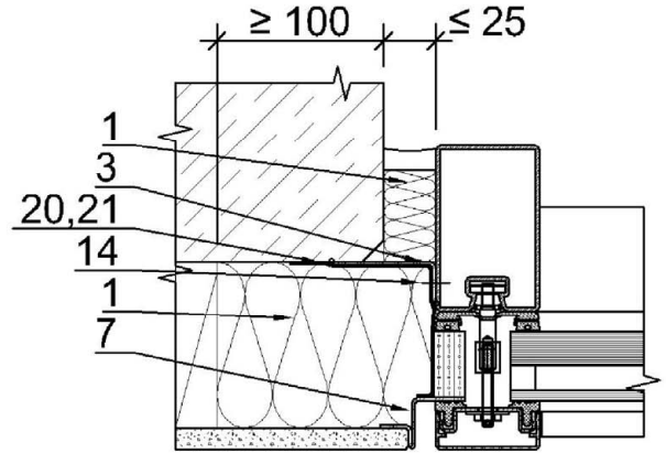
Schnitt 4.2.0.4
