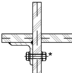
Schnitt 5.1.2.1
