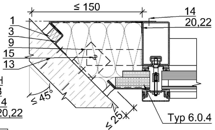
Schnitt 4.2.3.2
