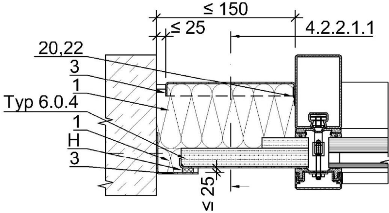
Schnitt 4.2.2.1.1
