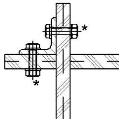
Schnitt 5.1.2.5
