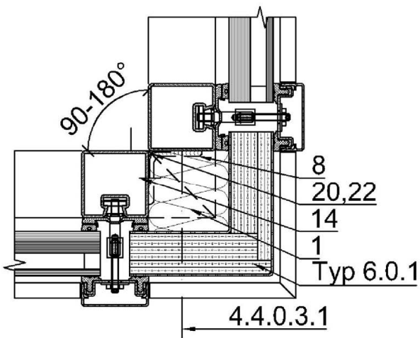
Schnitt 4.4.0.3
