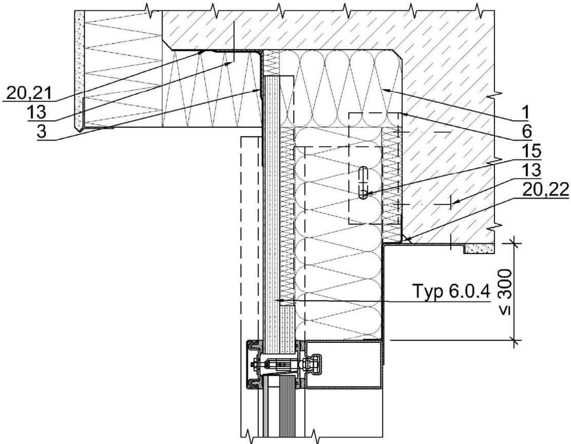
Schnitt 4.1.2.1
