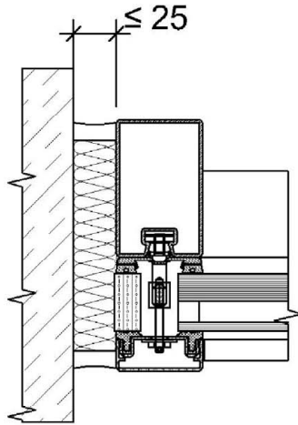
Schnitt 4.2.0.1
