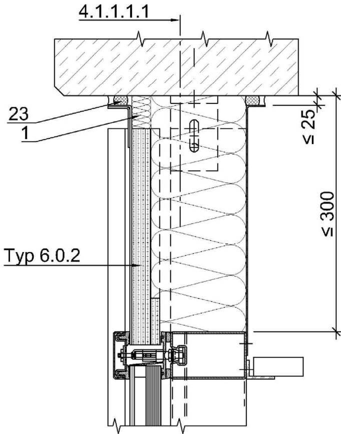
Schnitt 4.1.1.1
