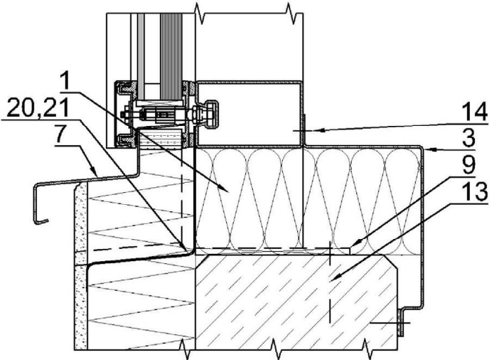
Schnitt 4.0.1.1
