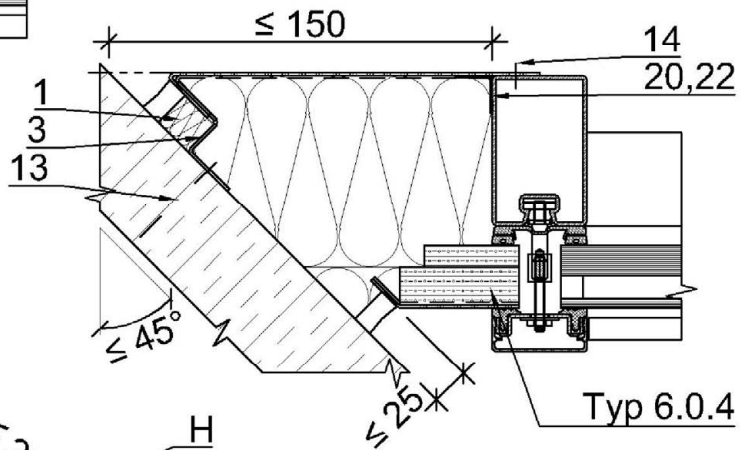
Schnitt 4.2.3.3
