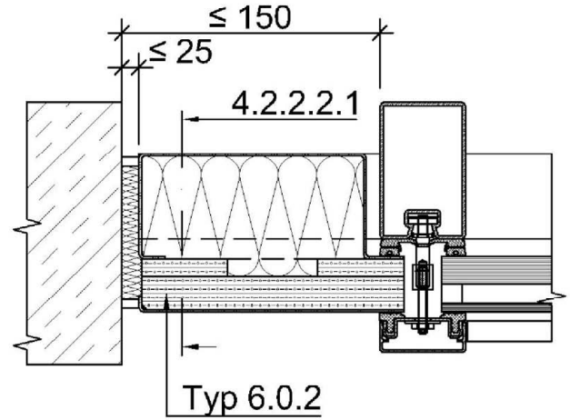
Schnitt 4.2.2.2
