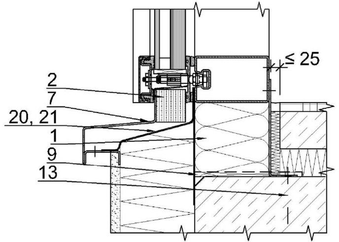
Schnitt 4.0.0.2
