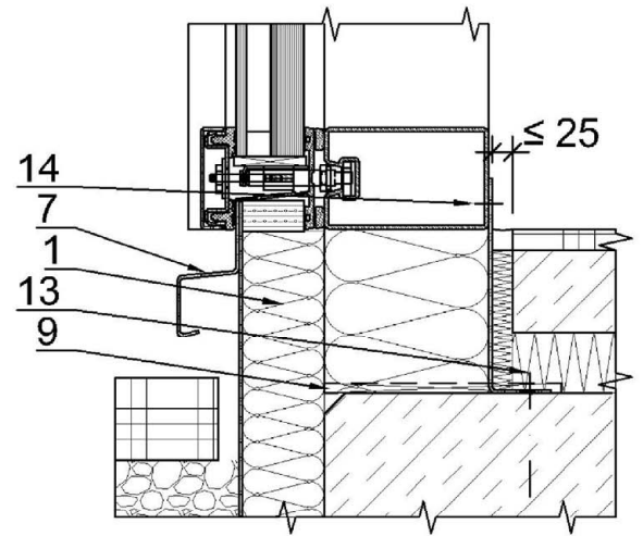
Schnitt 4.0.0.4
