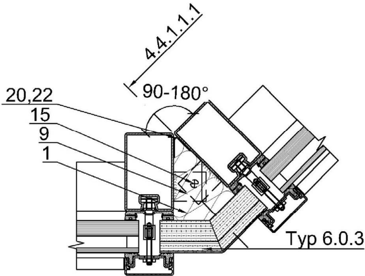
Schnitt 4.4.1.1
