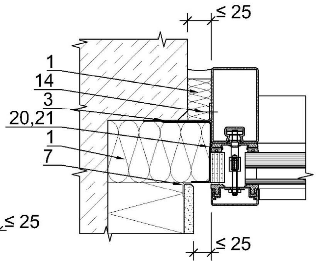
Schnitt 4.2.0.4
