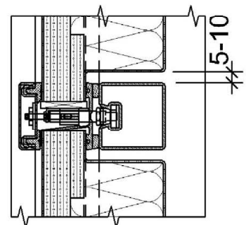
Schnitt 4.2.2.2.1
