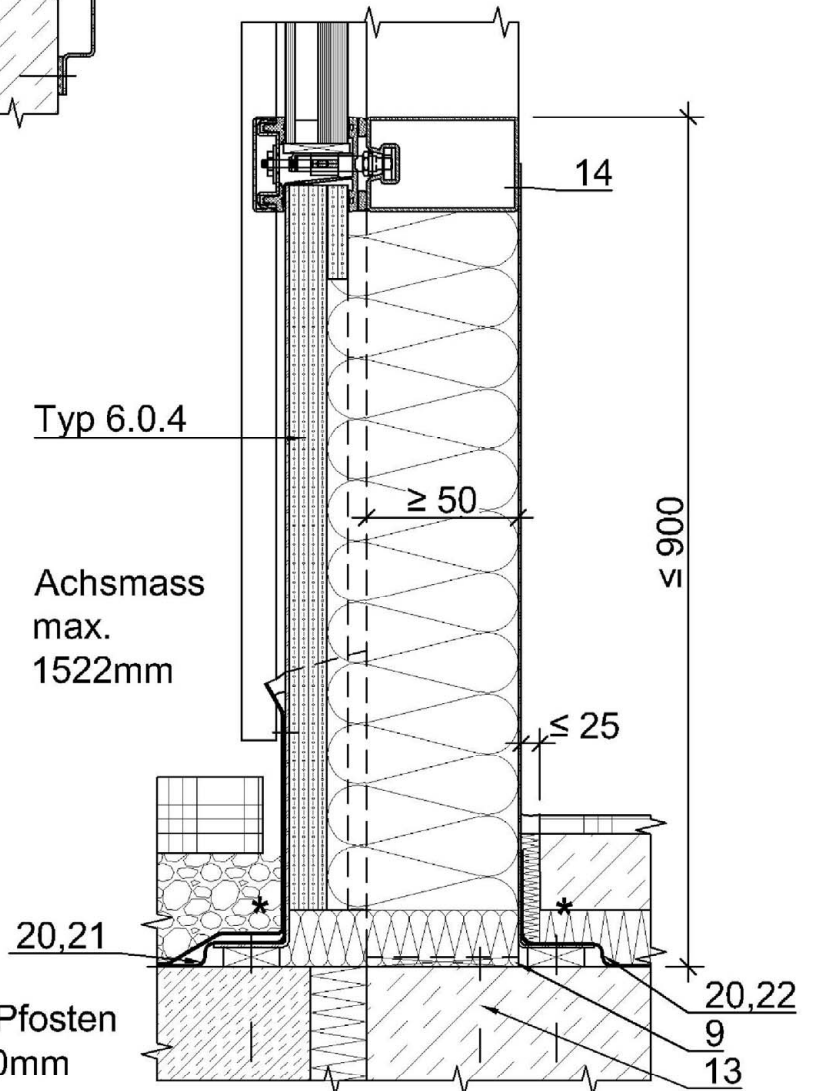
Schnitt 4.0.1.2
