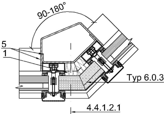
Schnitt 4.4.1.2
