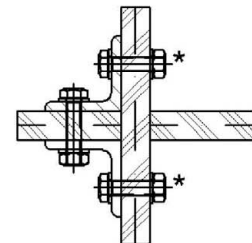
Schnitt 5.1.2.6
