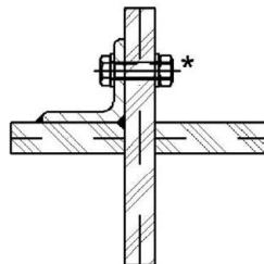
Schnitt 5.1.2.2
