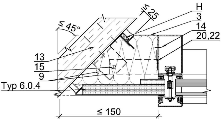
Schnitt 4.2.3.4
