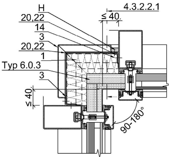
Schnitt 4.3.2.2
