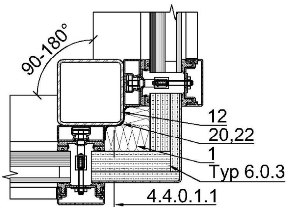
Schnitt 4.4.0.3
