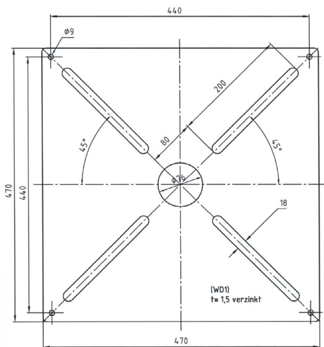
Hitzeschild für Spin Flachdachablauf aus Edelstahl 0153.74.15
