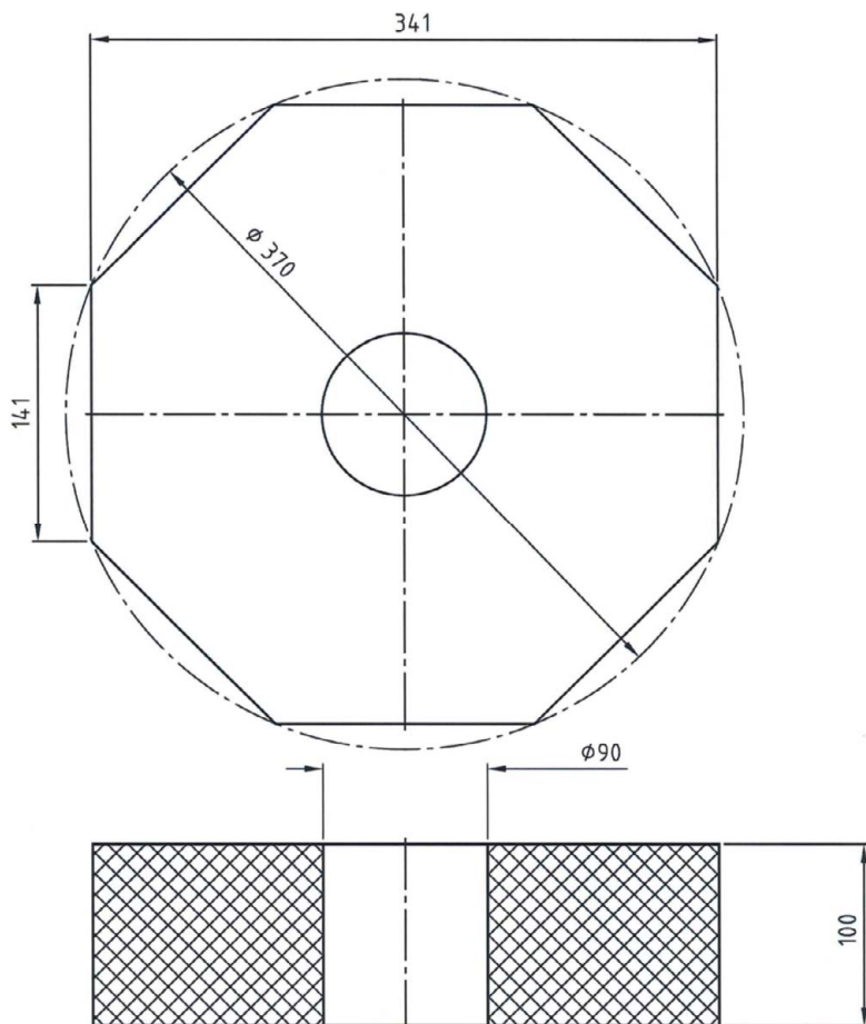
Isolierkörper aus Schaumglas für Spin Flachdachablauf aus Edelstahl 0150.12.69
