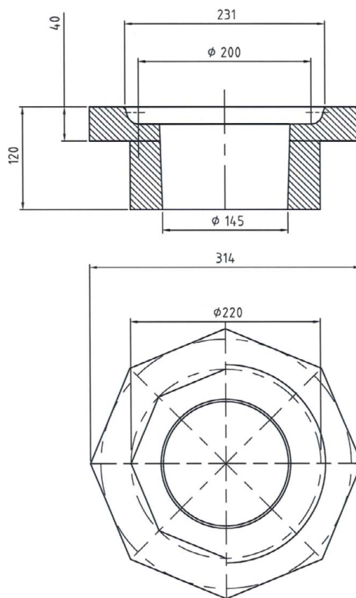
Isolierkörper aus Schaumglas für Spin Flachdach- ablauf aus Gusseisen 7040.22.00
