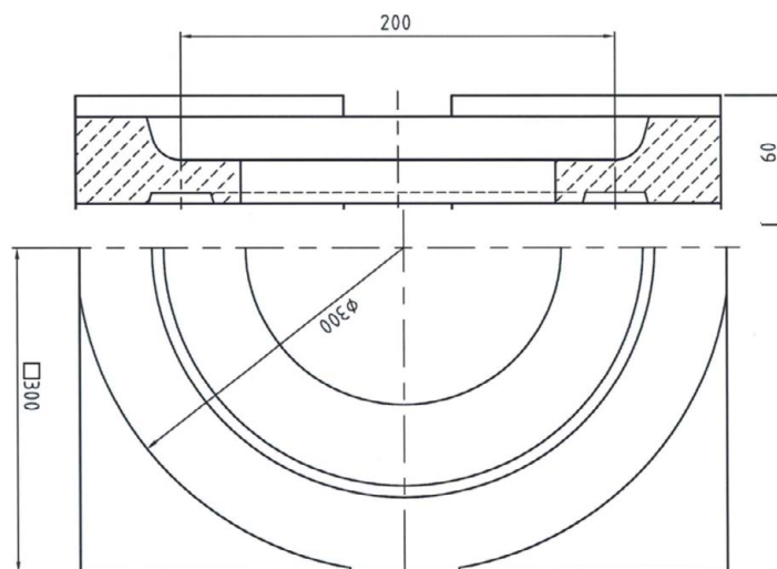
Isolierkörper aus Schaumglas für Spin Flachdach- ablauf aus Gusseisen 7040.12.00
