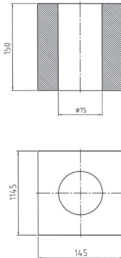
Mineralwolle-Rohrschale für Spin Fachdachablauf aus Edelstahl 0174.46.57
