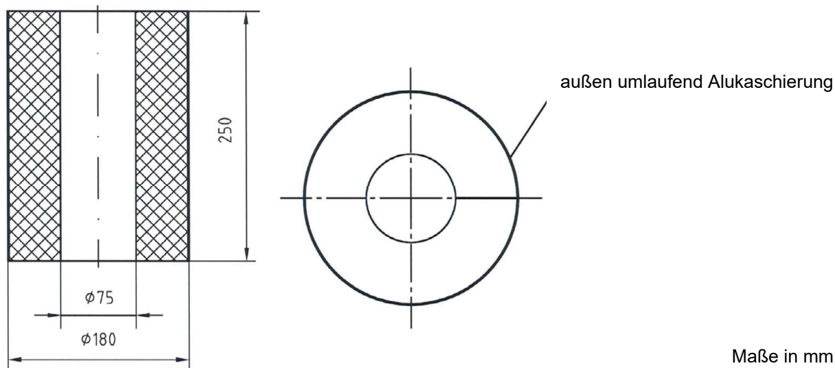
Mineralwolle-Rohrschale für Spin Fachdachablauf aus Edelstahl 0174.46.57
