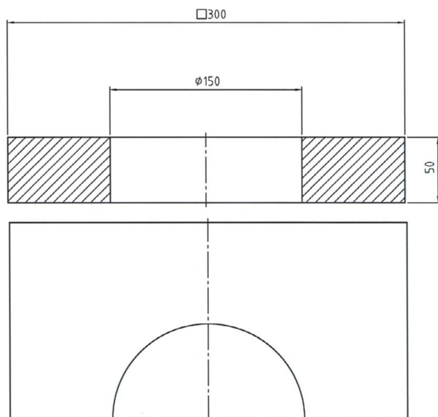
Isolierkörper aus Schaumglas für Spin Flachdach- ablauf aus Gusseisen 7040.02.00
