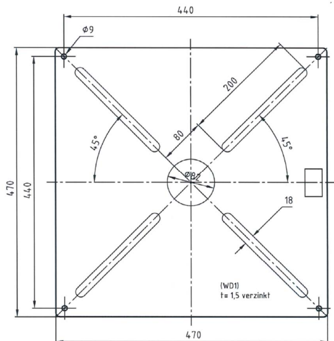
Hitzeschild für Spin Flachdachablauf aus Gusseisen 5169.20.17
