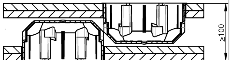
Anordnung beidseitig neben- oder übereinander, beidseitig der Wand versetzt
