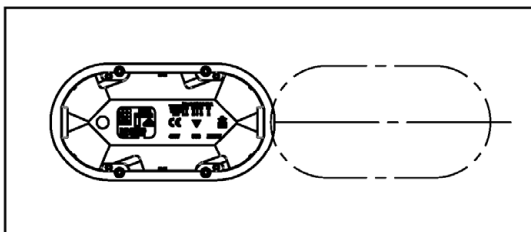
Holzrippe (Kantholz 60x40)
