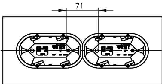
Anordnung einseitig neben- oder übereinander (Zweifachkombination)
