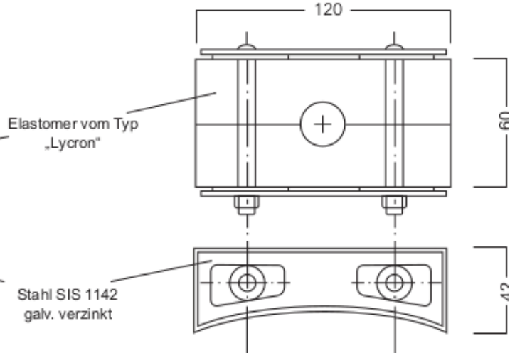
Schlussdichtung STG-2
