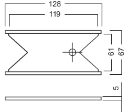
Ankerscheibe
