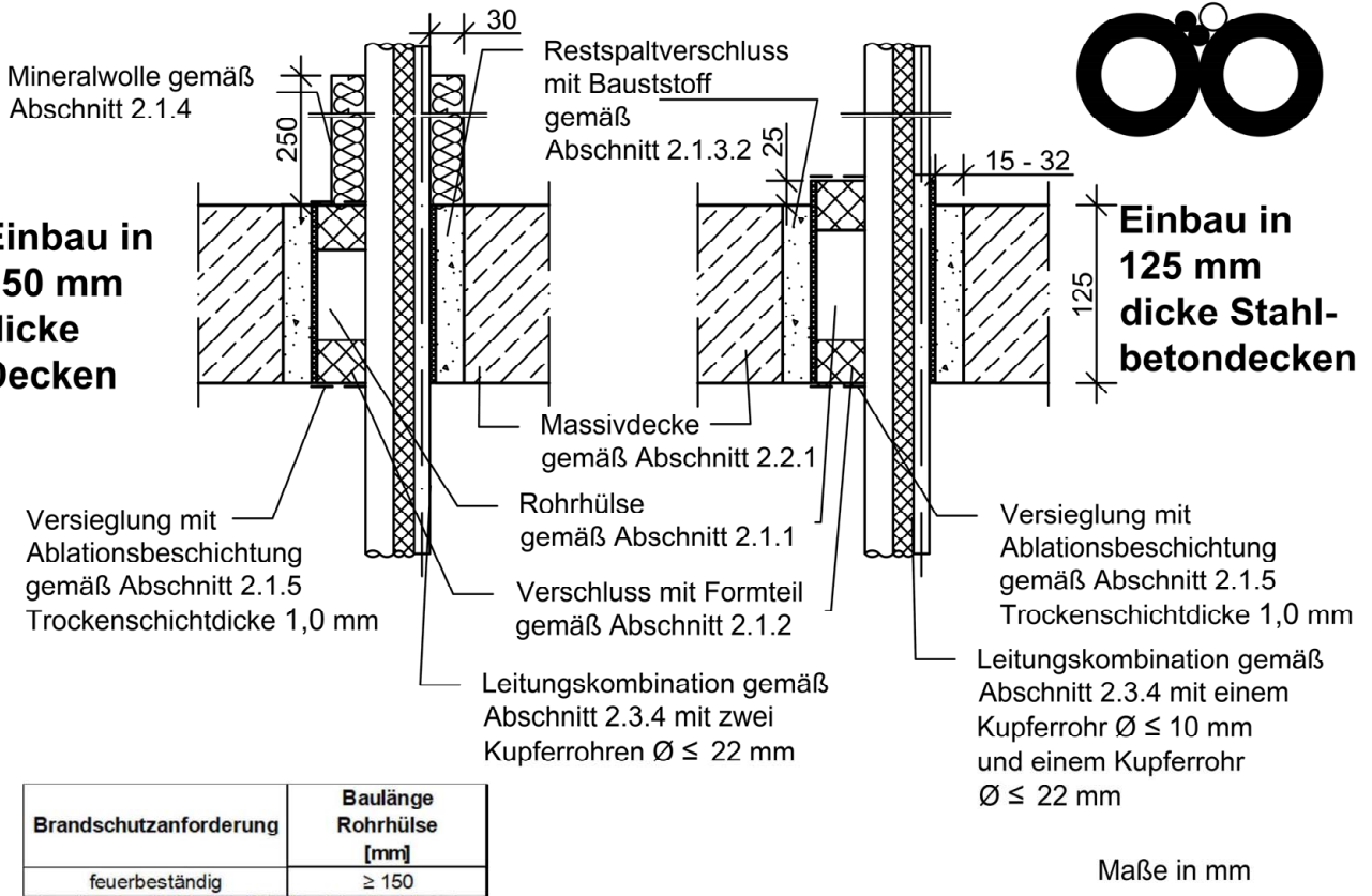
Ansicht Leitungskombinationen
