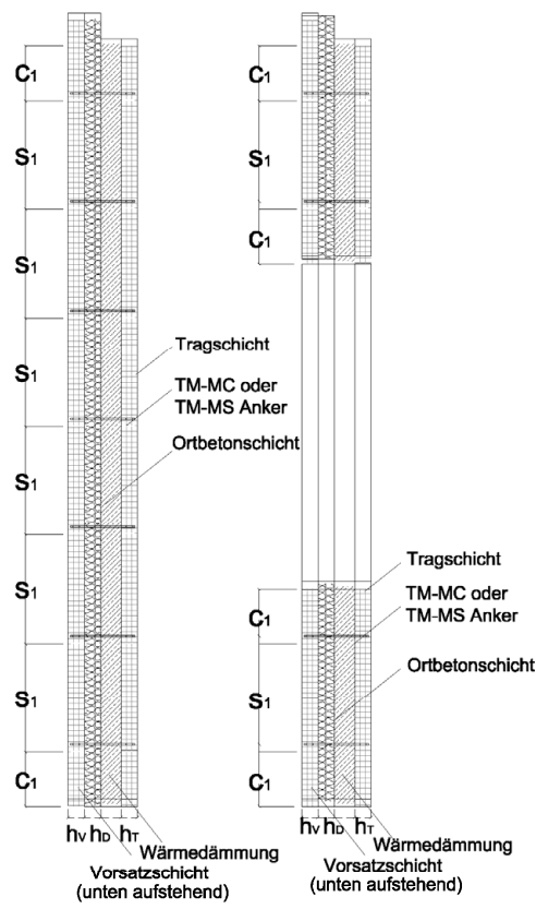
Sandwichwand Seitenansicht
