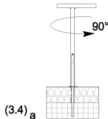
(3.4) a TM-MC bzw. TM-MS Anker um 90° drehen
