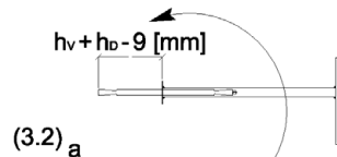
(3.2) a TM-MC bzw. TM-MS Anker und Setzhilfe hochstellen
