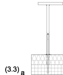
(3.3) a TM-MC bzw. TM-MS Anker bis zum Anschlag einsetzen
