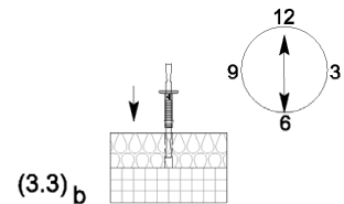
(3.3) b TM-MC bzw. TM-MS Anker bis zum Anschlag einsetzen
