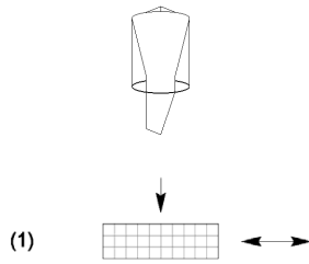
(1) Beton der Vorsatzschicht einfüllen und verdichten
