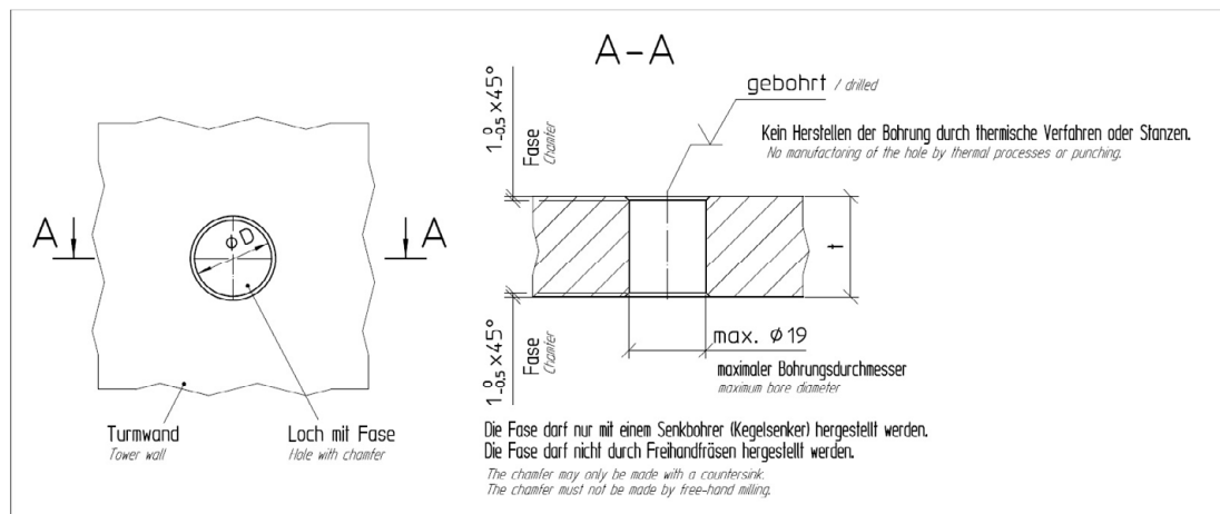
Abbildung 2 - Detail Bohrungen in Mantelblechen
