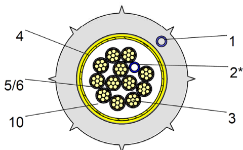
Schnitt A-A (innerhalb L_{tr} )
