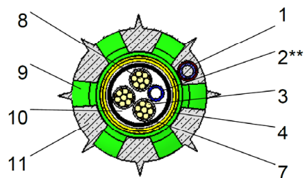
Schnitt B-B (innerhalb L_{tb} )
