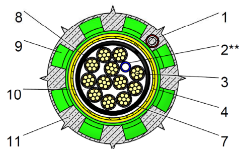
Schnitt B-B (innerhalb L_{tb} )
