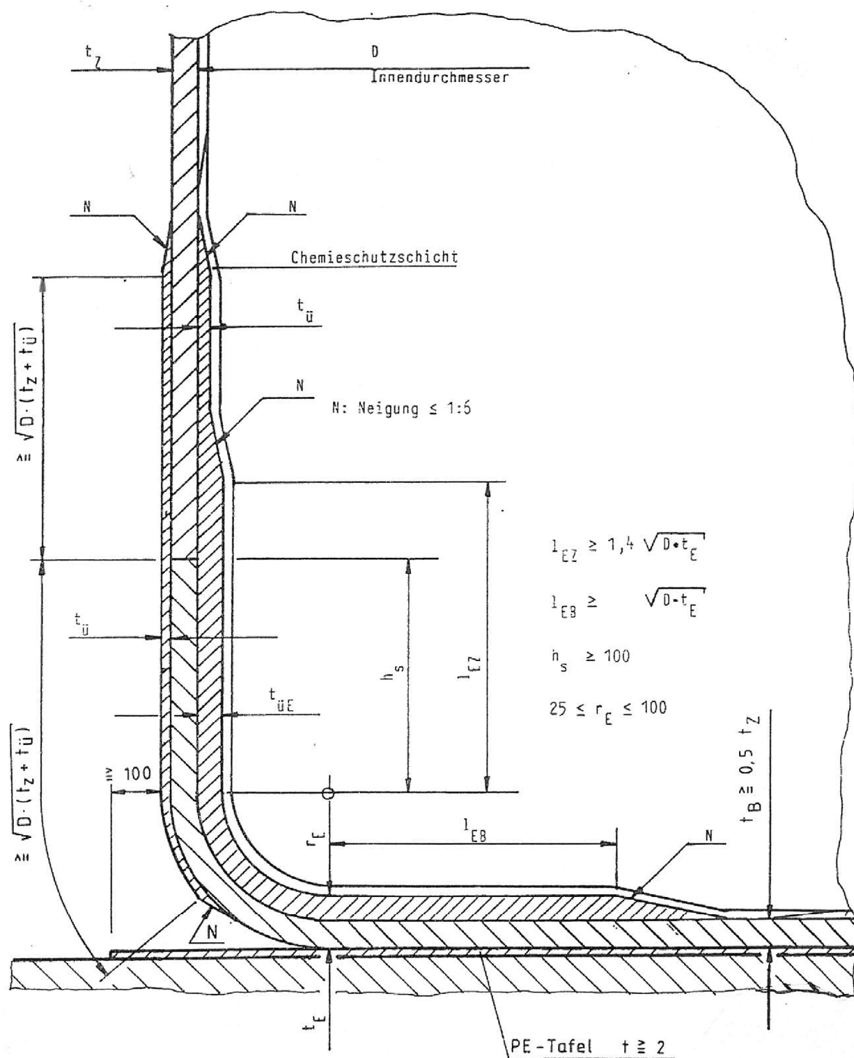
Flachbodenbehälter aus GF-UP/GF-PHA mit innerer Vlies- bzw. Chemieschutzschicht
