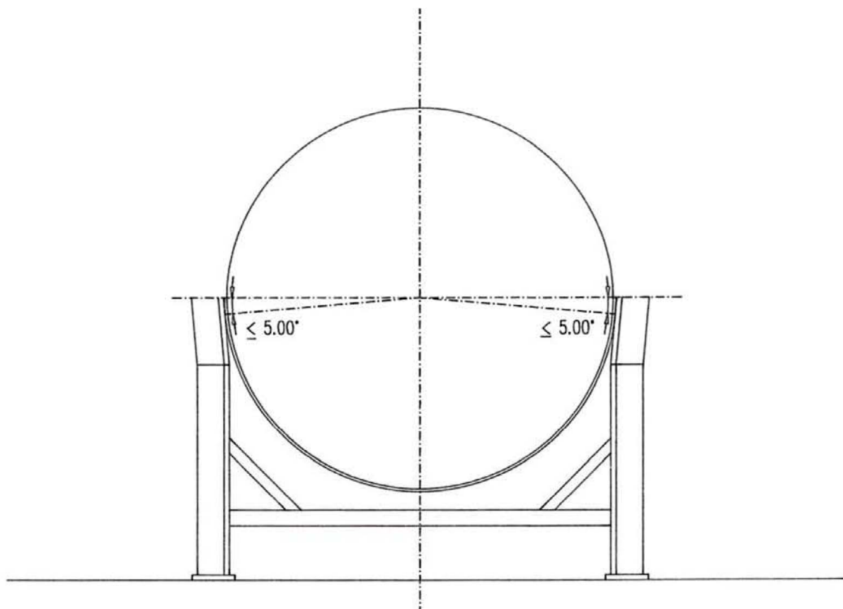
STAHLBAND MIT STUTZEN ÜBER UMSCHLINGUNGSWINKEL < 5^\circ VERSCHWEIBT
