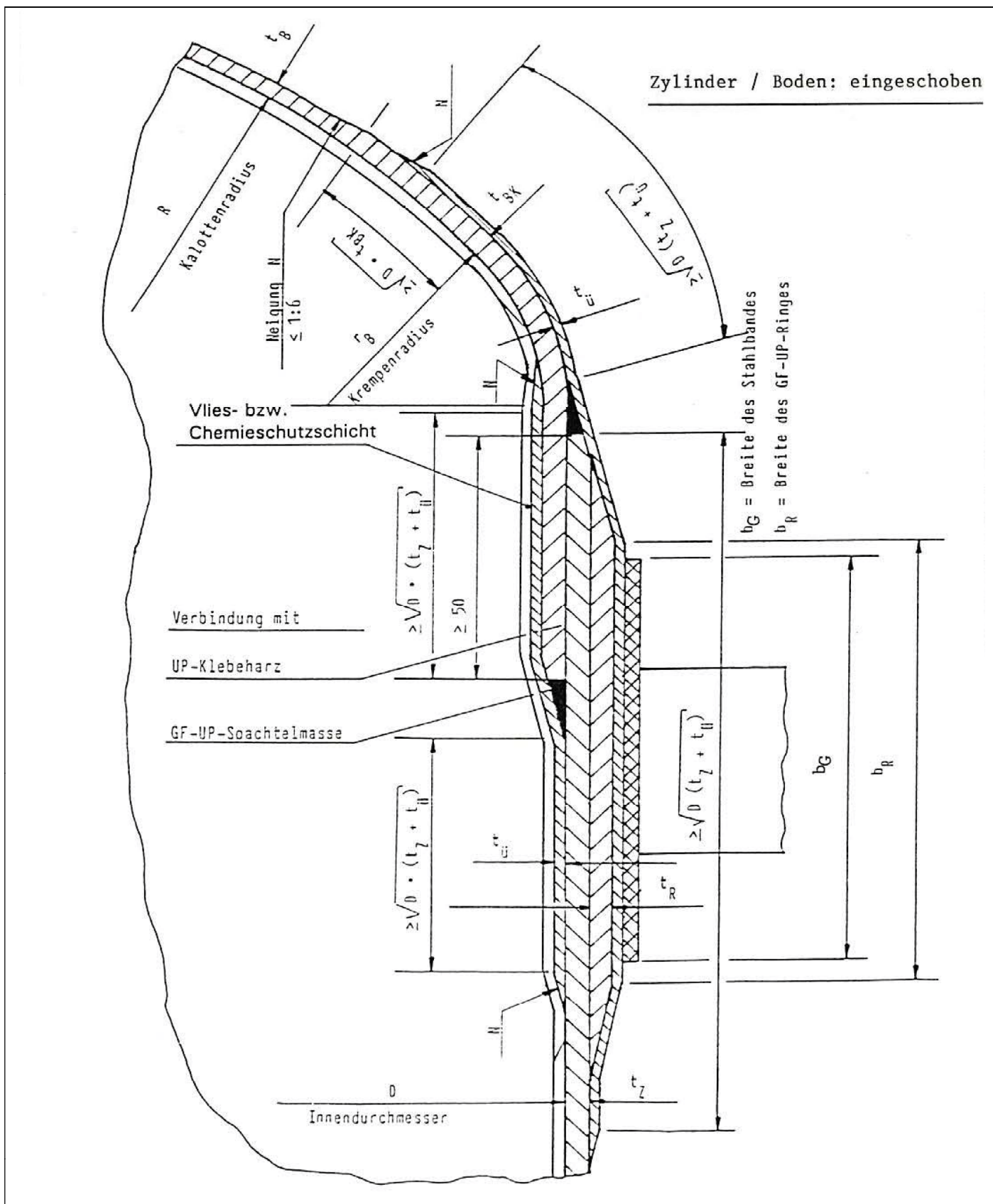
Liegende Behälter aus GFK mit innerer Vliesschicht oder Chemieschutzschicht im Übergangsbereich Versteifungsring
