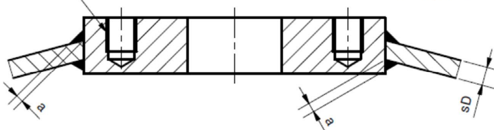
Variante 2 für Kegeldach
