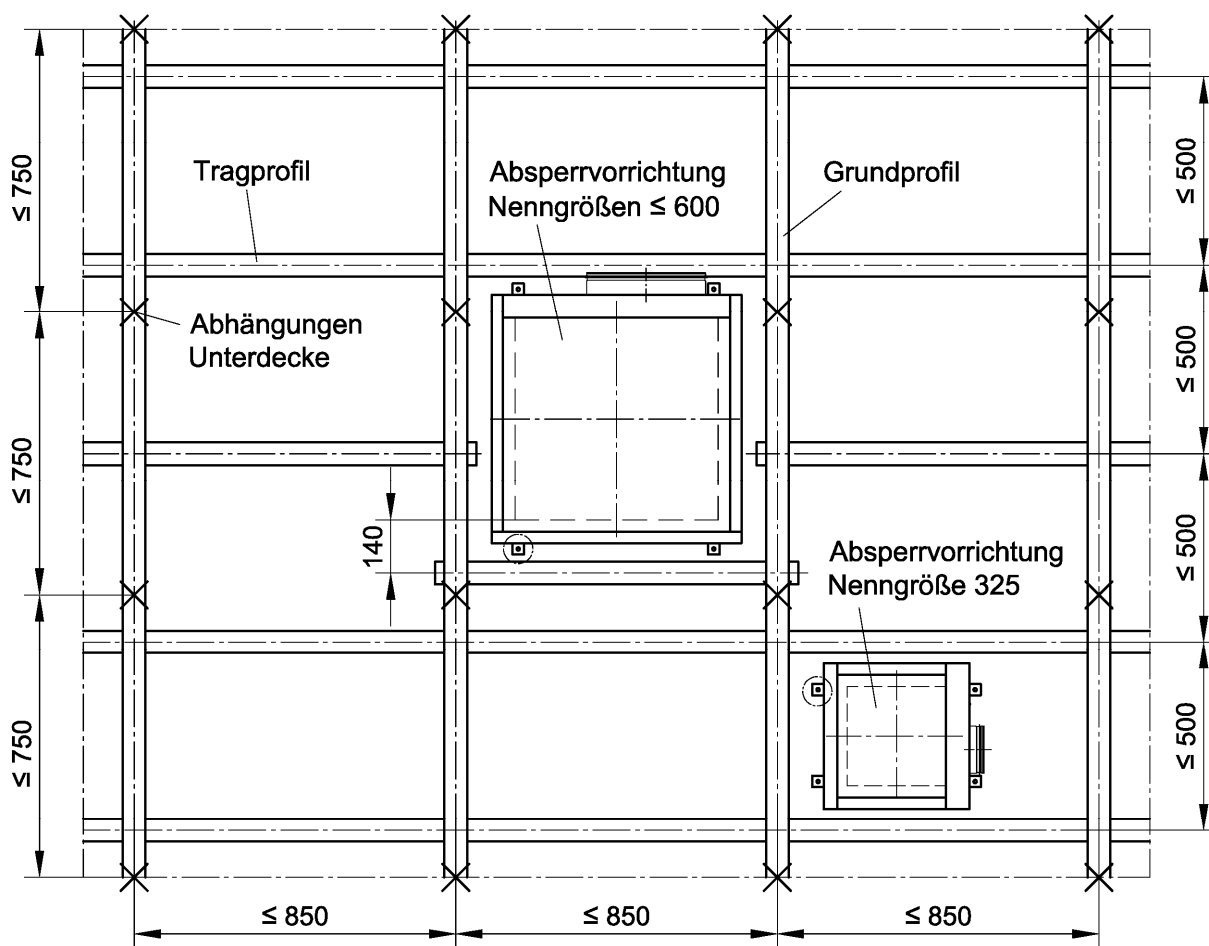
Abhängung der Absperrvorrichtungen
