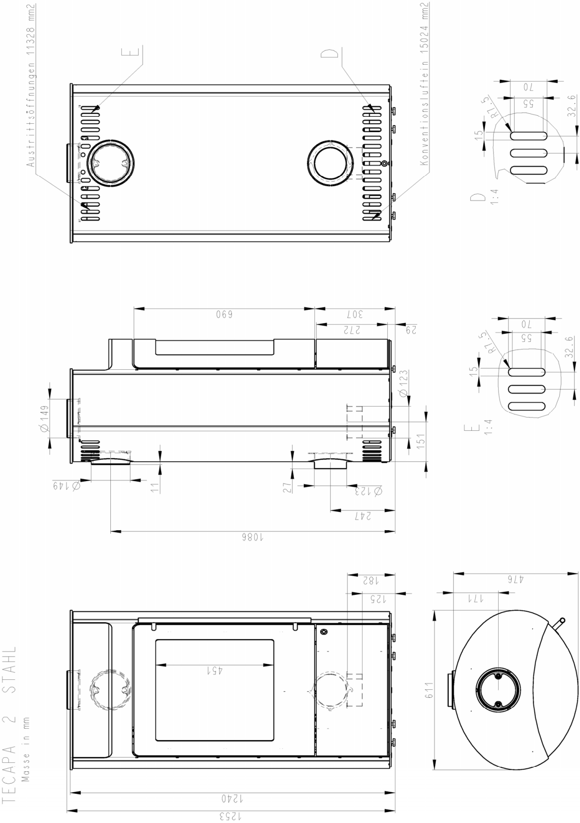
Raumluftunabhängige Kaminöfen in verschiedenen Ausführungen
