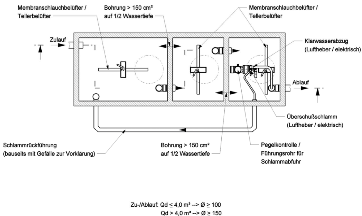
Draufsicht ohne Abdeckung
