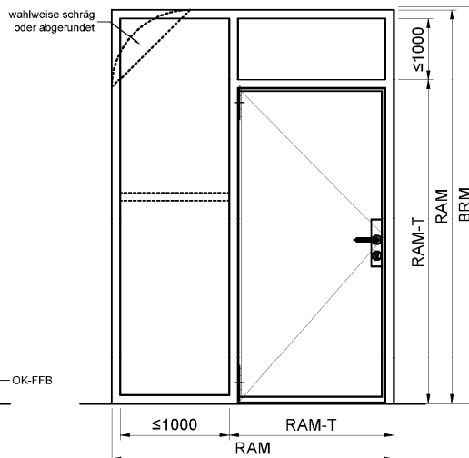
Tür mit Holzblockzarge oder Rohrrahmenzarge und Seitenteil / Oberteil
