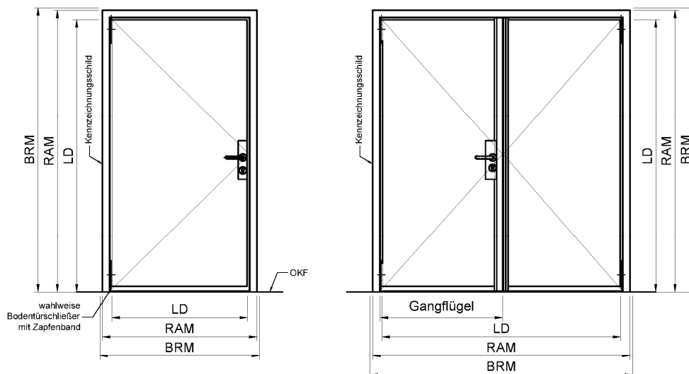
Dargestellt Gangflügel DIN links Gangflügel DIN rechts - spiegelbildlich
