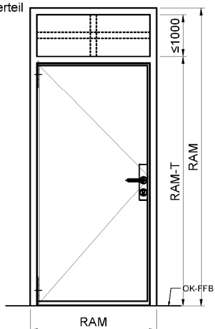
Tür mit Holzblockzarge oder Rohrrahmenzarge und Oberteil Tür mit Holzblockzarge oder Rohrrahmenzarge und Seitenteil(en) / Oberteil
