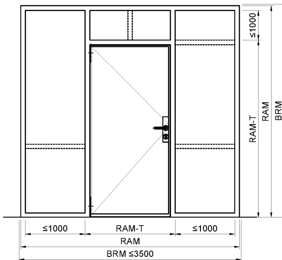
Tür mit Holzblockzarge oder Rohrrahmenzarge und Oberteil Tür mit Holzblockzarge oder Rohrrahmenzarge und Seitenteil(en) / Oberteil
