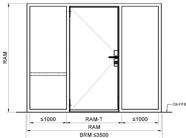
Tür mit Holzblockzarge oder Rohrrahmenzarge und Oberteil Tür mit Holzblockzarge oder Rohrrahmenzarge und Seitenteil(en) / Oberteil
