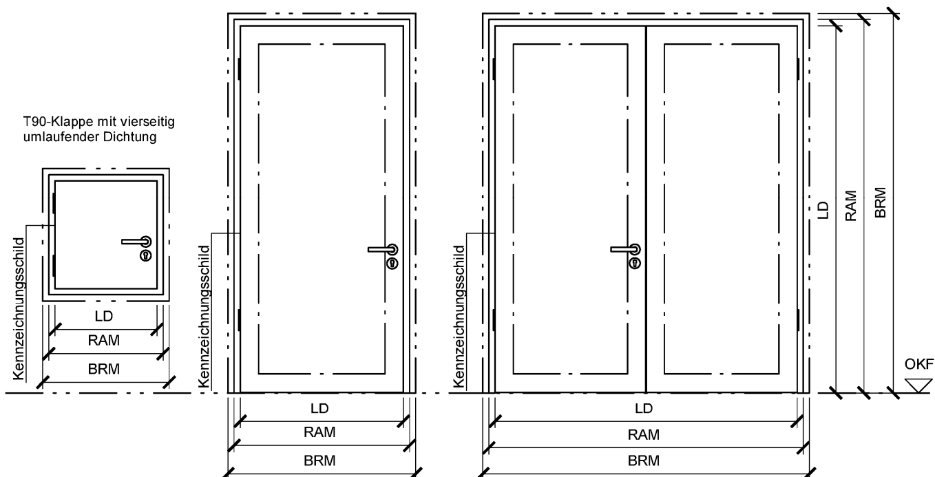
Darstellung: Gangflügel DIN links; Gangflügel DIN rechts spiegelbildlich
