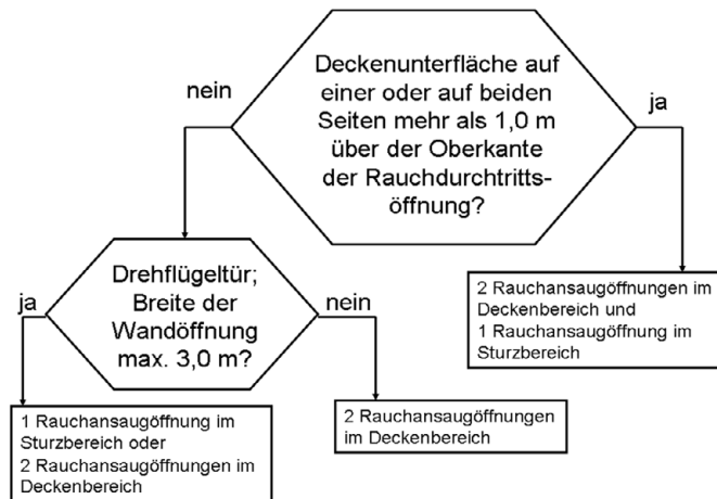
Bild 6: Entscheidungsdiagramm
