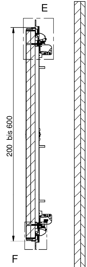
Schnitt D-D
